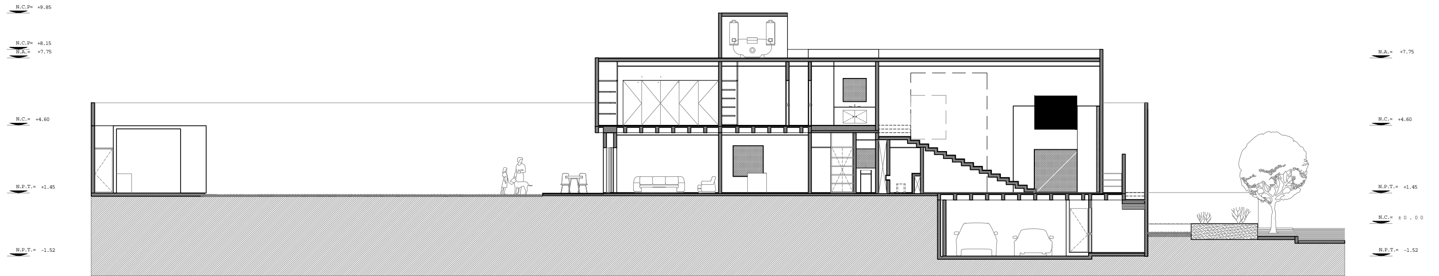
CORTE C-C'
