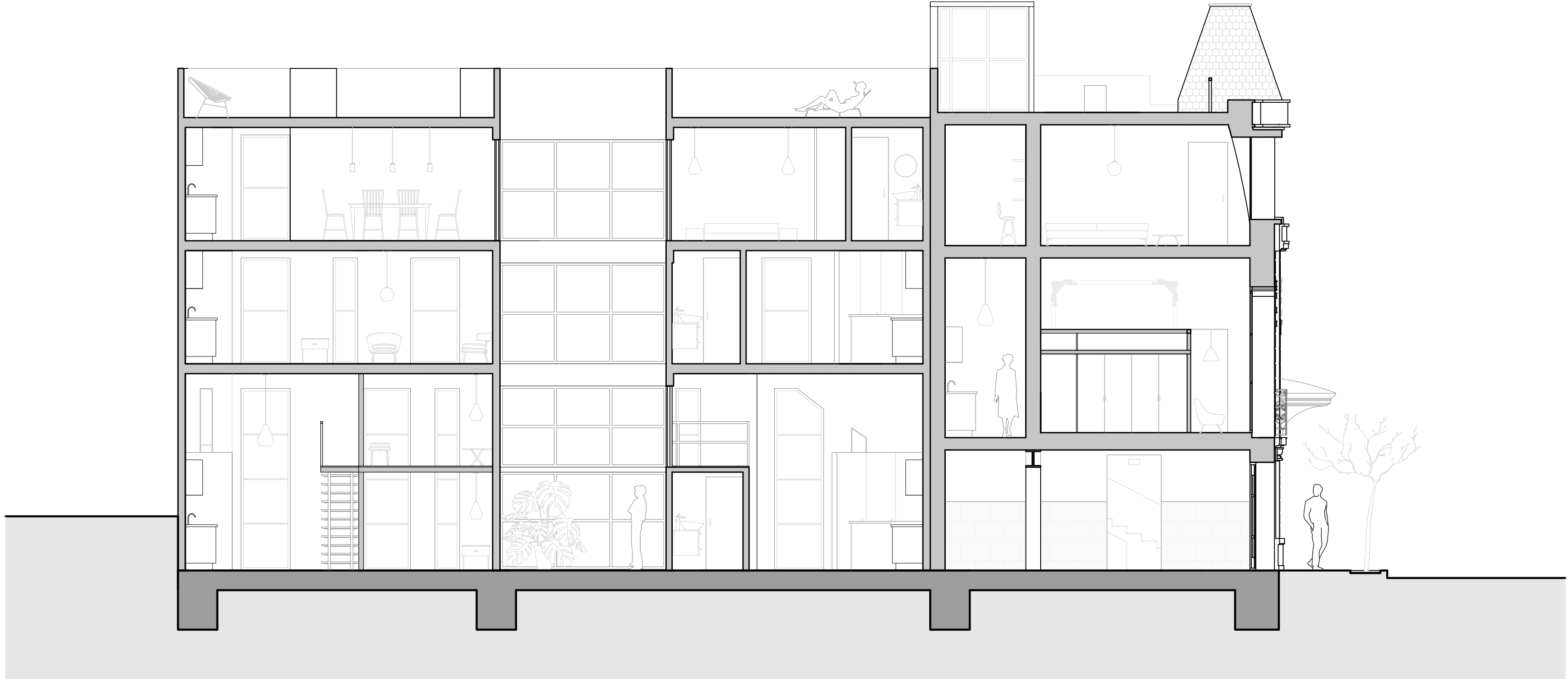
MM34 | MAR MEDITERRANEO 34 SECCIÓN LONGITUDINAL | LONGITUDINAL SECTION
