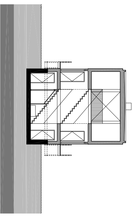
doorsnede B
