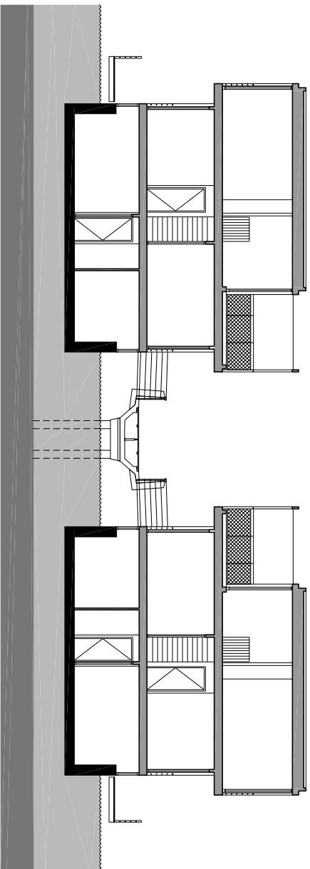
doorsnede A
