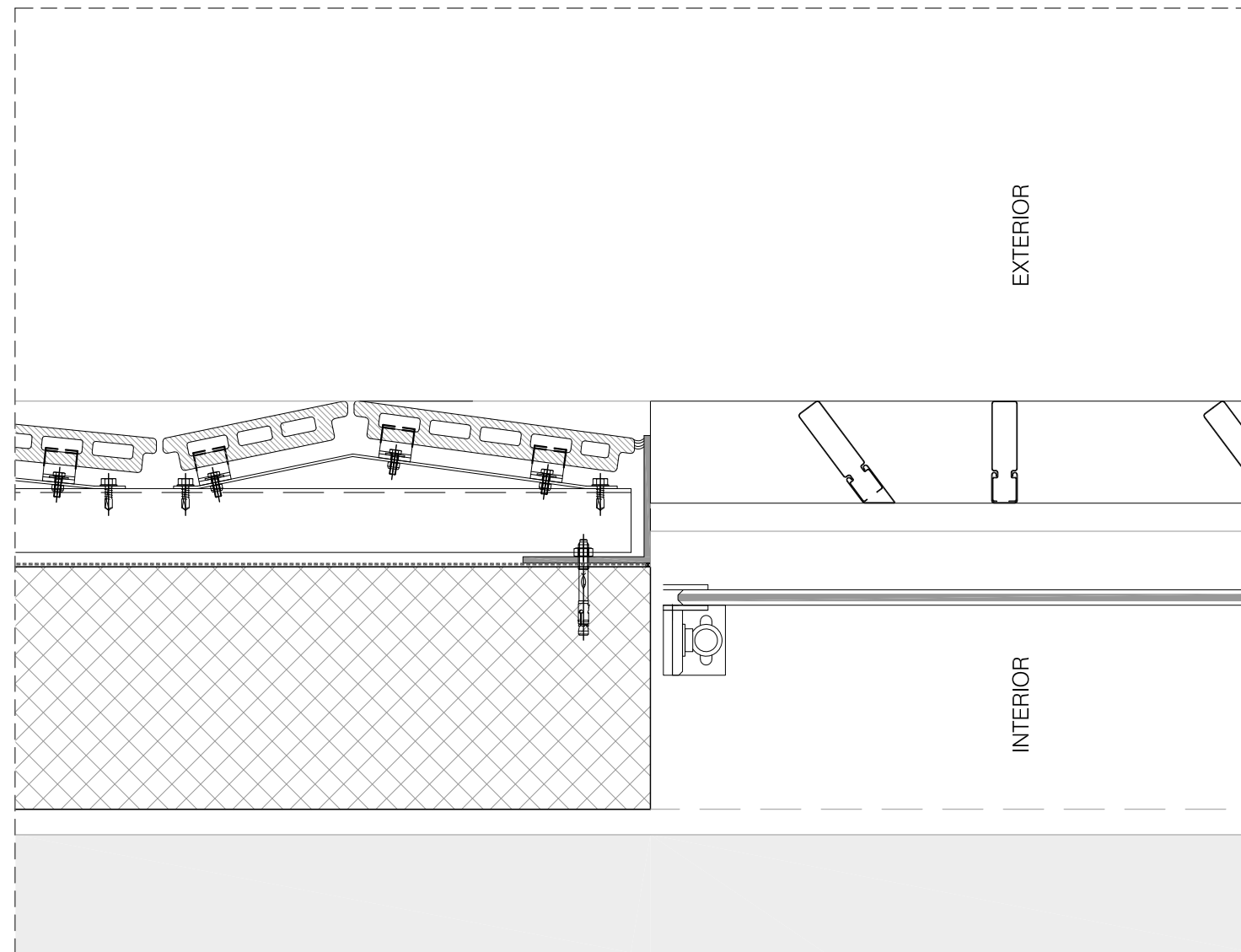
Detalle Planta fijación lamas
