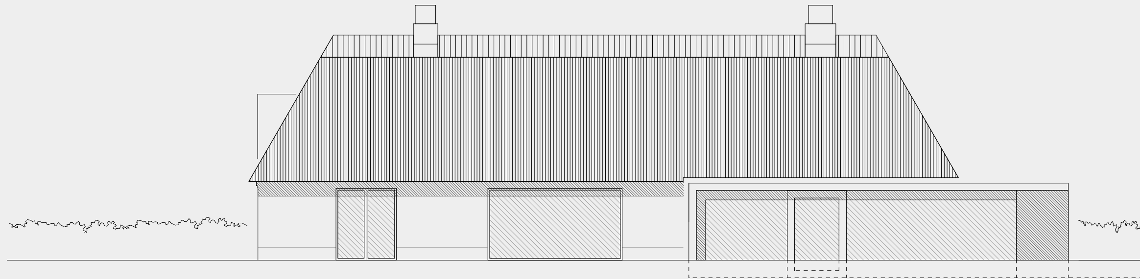
opstalt mod nord
