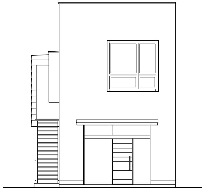
Elevation 1:100
