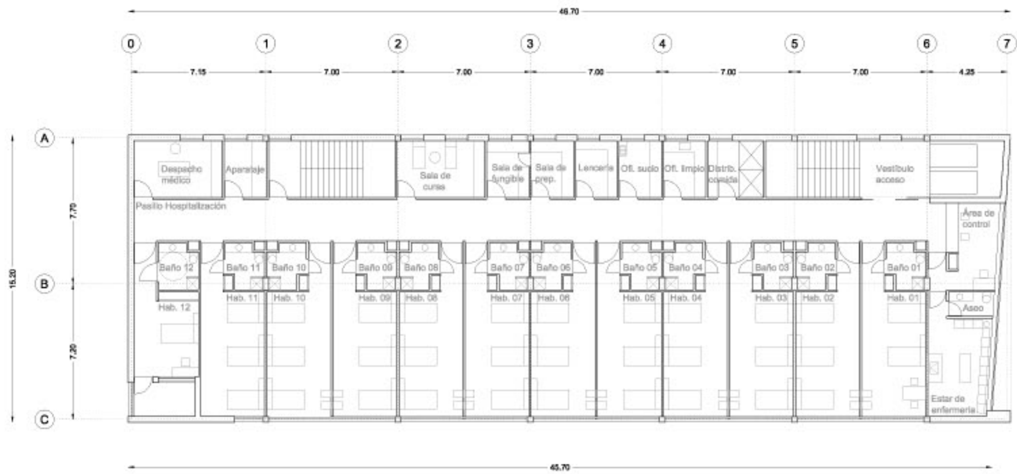
PLANTA TERCERA
