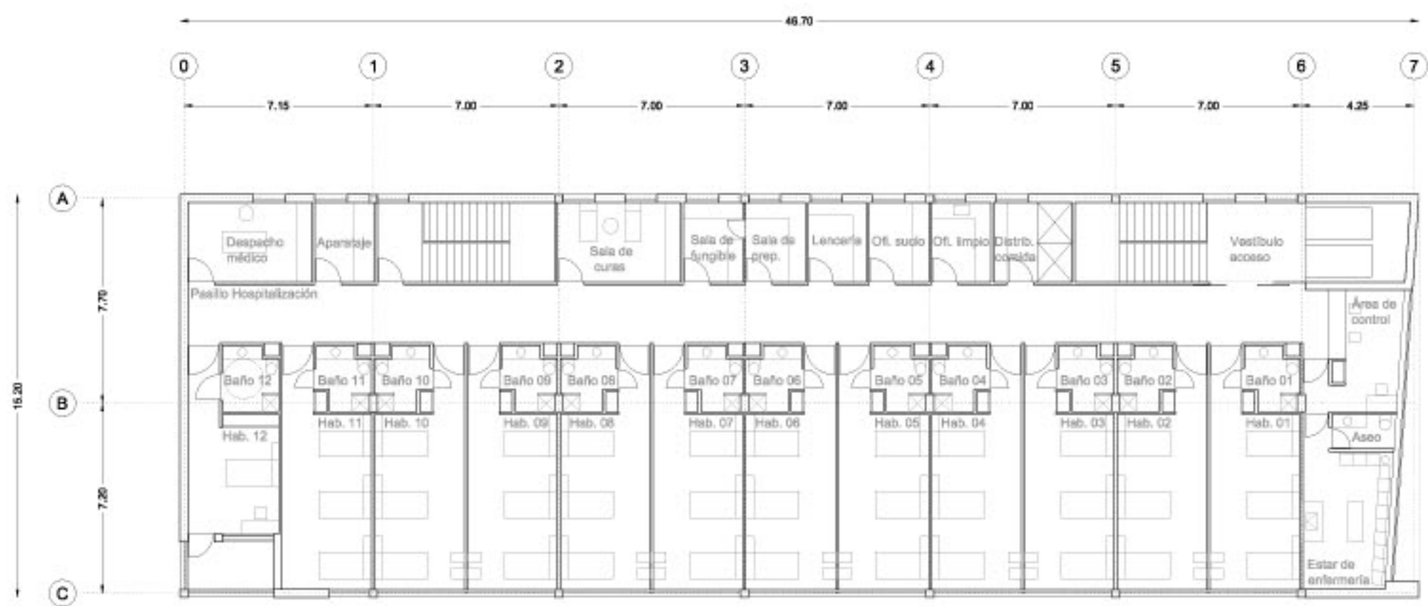
PLANTA CUARTA
