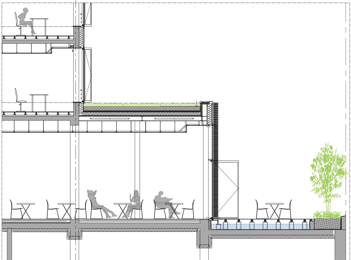
COUPE A-A
