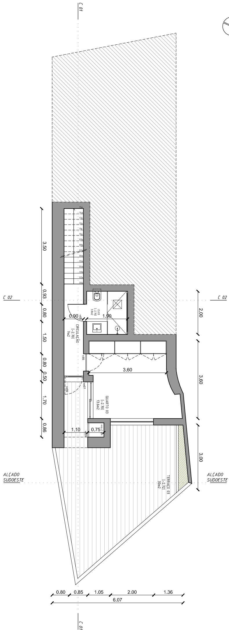
PROPOSTA - PLANTA DO PISO -1
