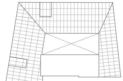
planta de cubiertas
