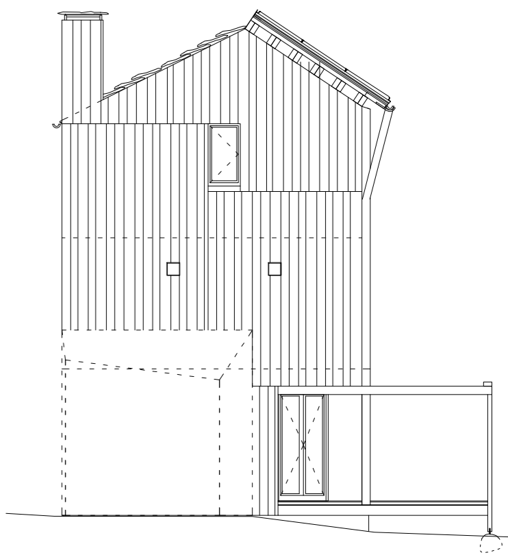
prospetto ovest/ west elevation
