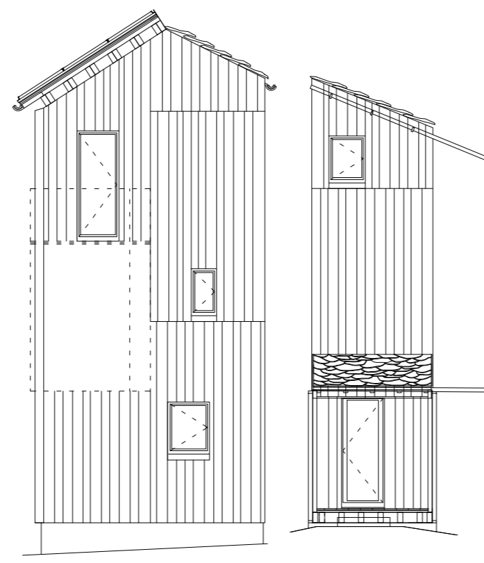
prospetti est/ east elevations
