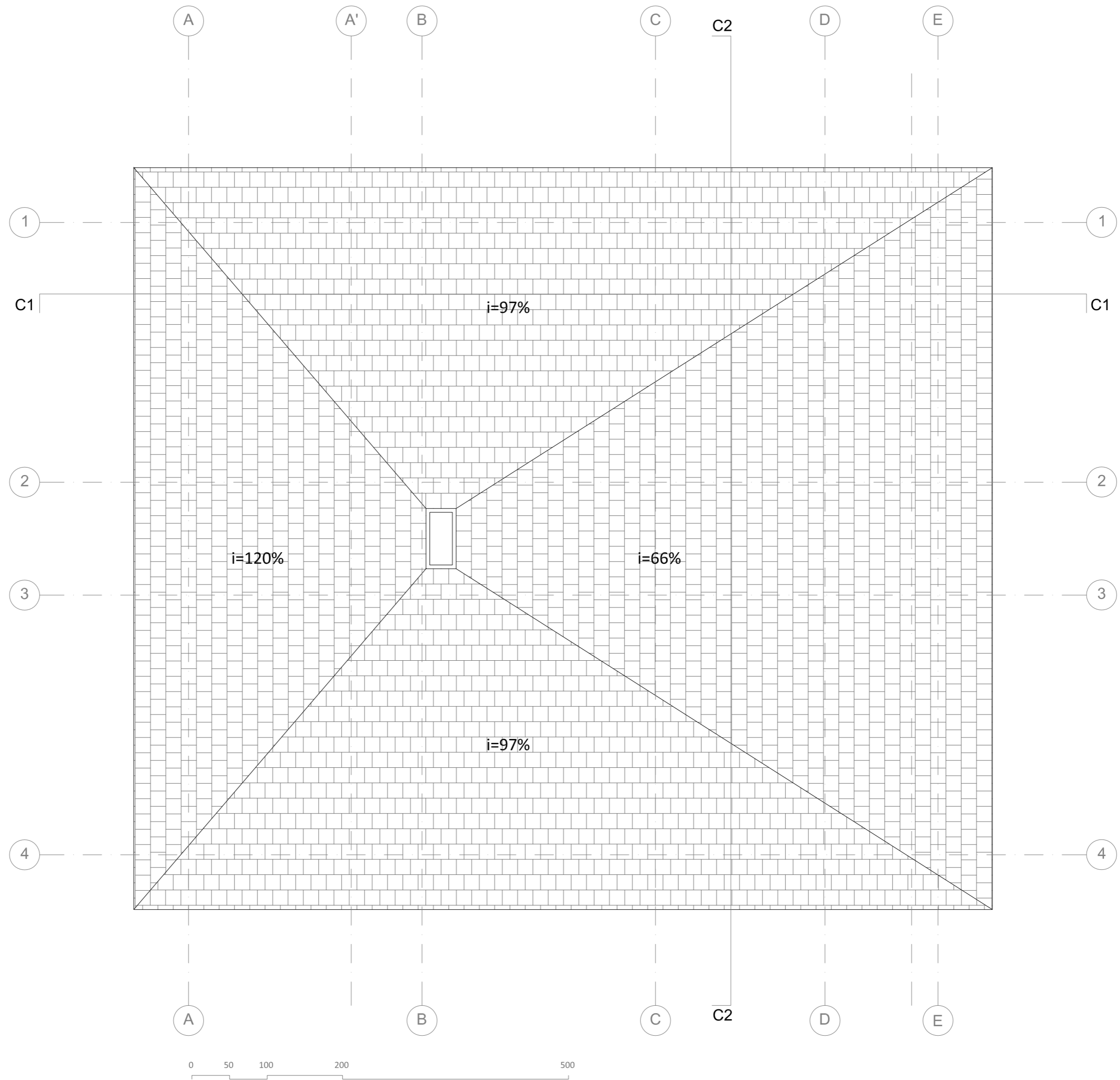
planta cubierta
