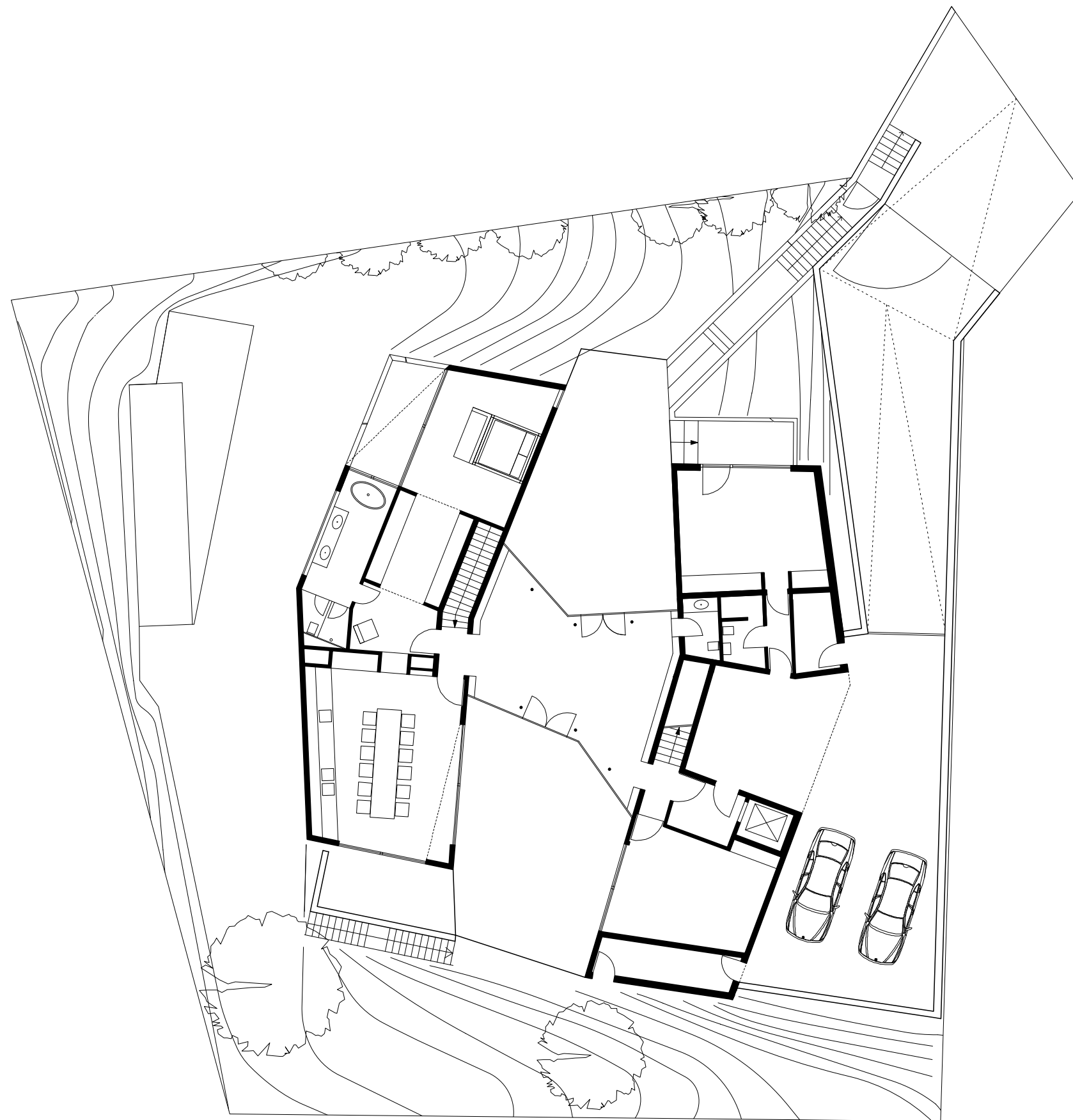
Erdgeschoss M 1:200
