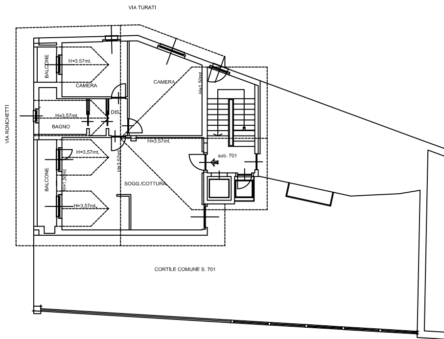
PIANO SECONDO
