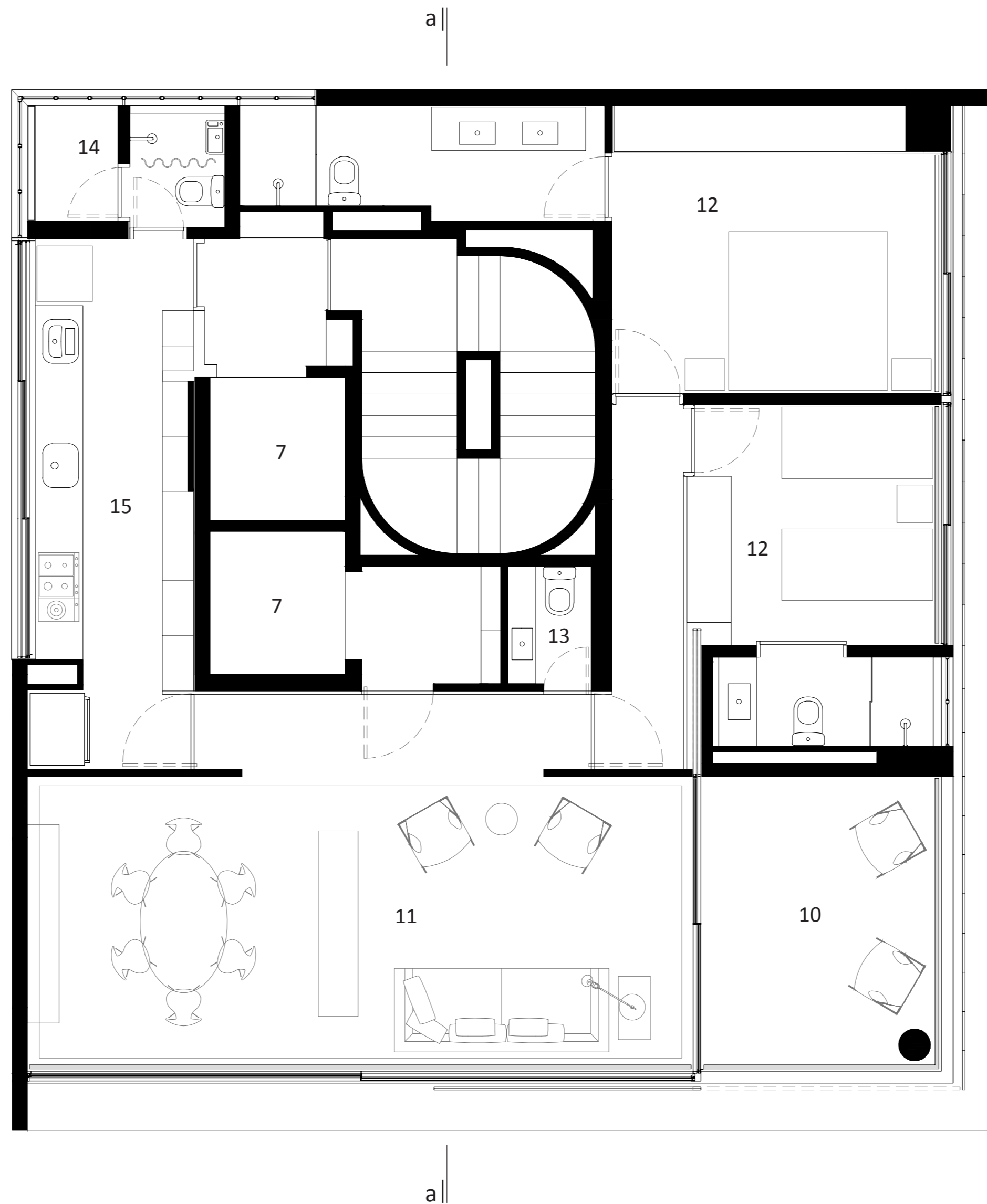
planta tipo _ type floor plan 1:50
