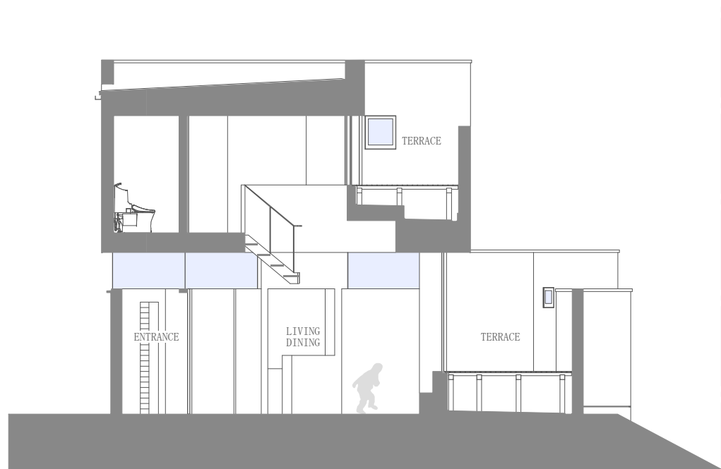
Section A-A' S=1:100
