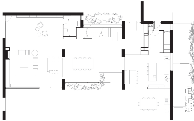
Planta Baja
