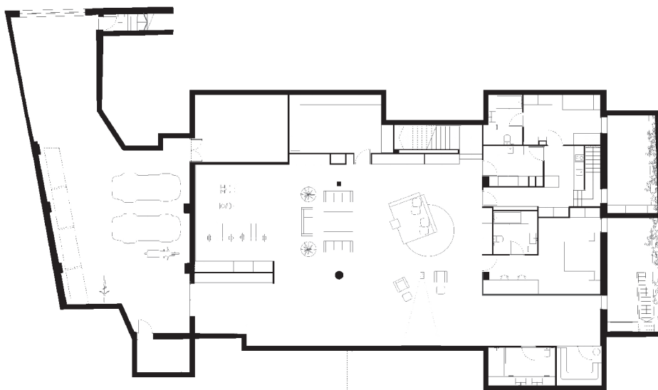
Planta Sótano
