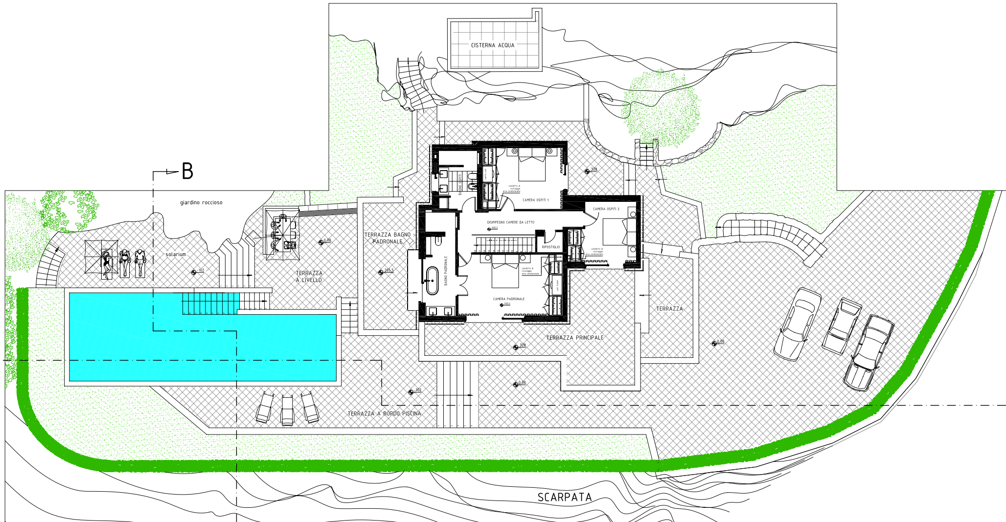
PIANTA DEL PIANO SUPERIORE - 1:100
