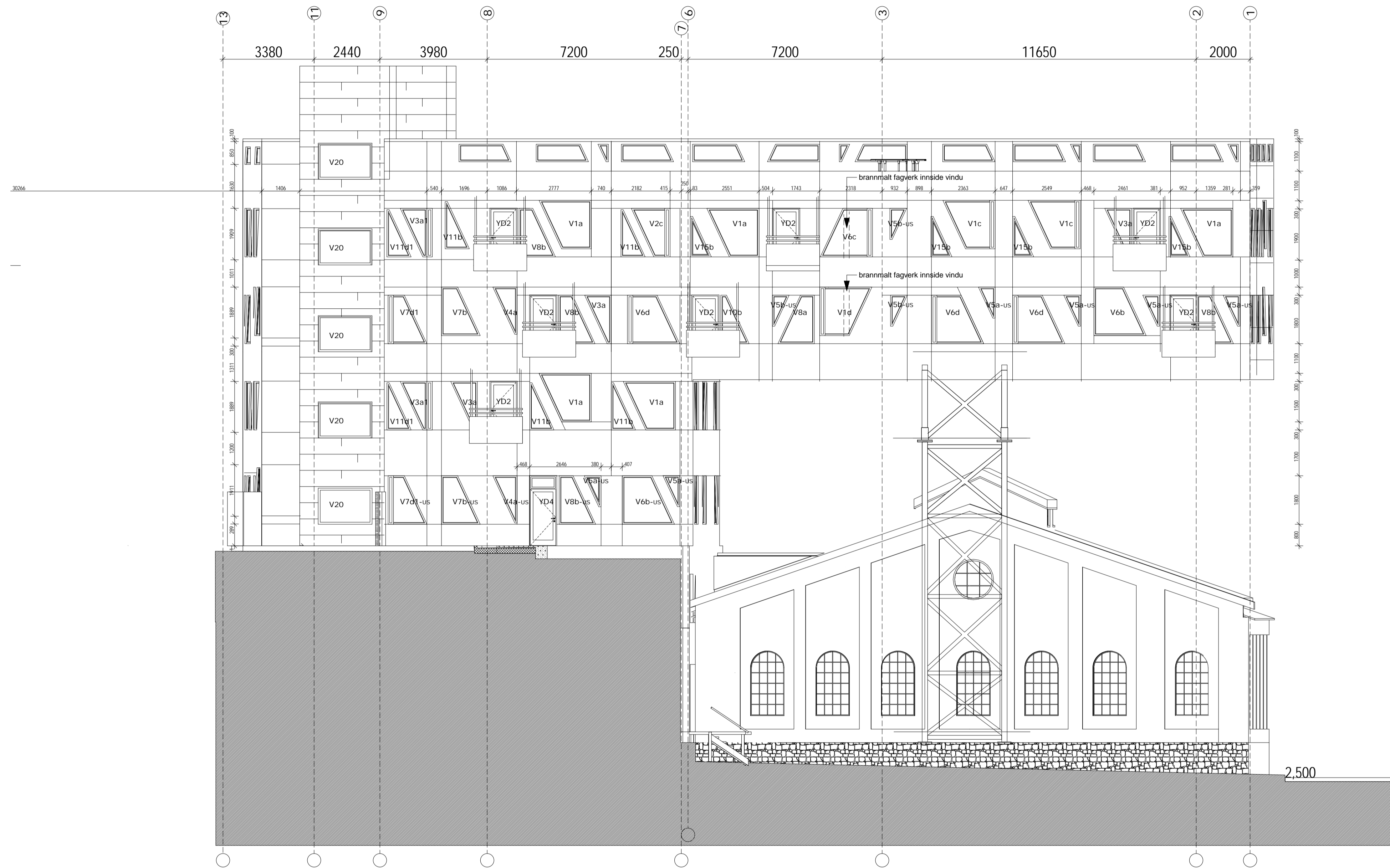
Strandlien hus C Fasade mot Verket Dato: 21.01.2014 LINK arkitektur AS
