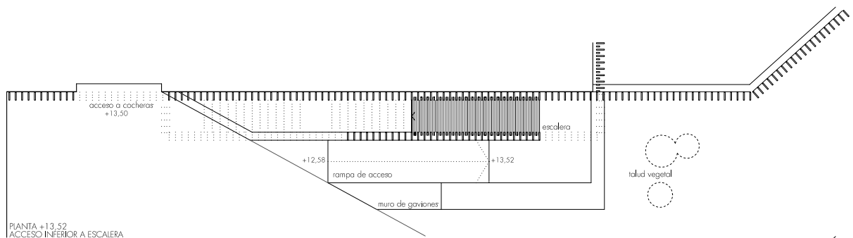
PIANTA +13,52 ACCESO INFERIOR A ESCALERA
