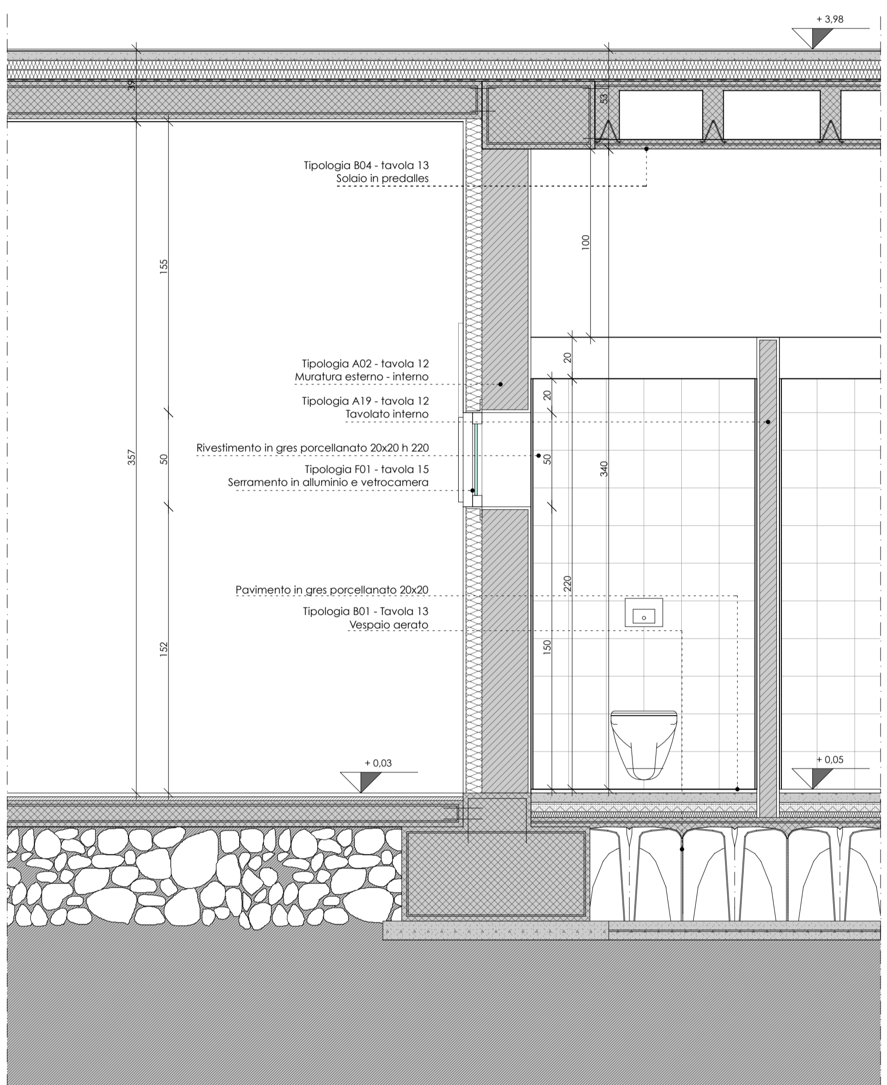
SEZIONE D-D
