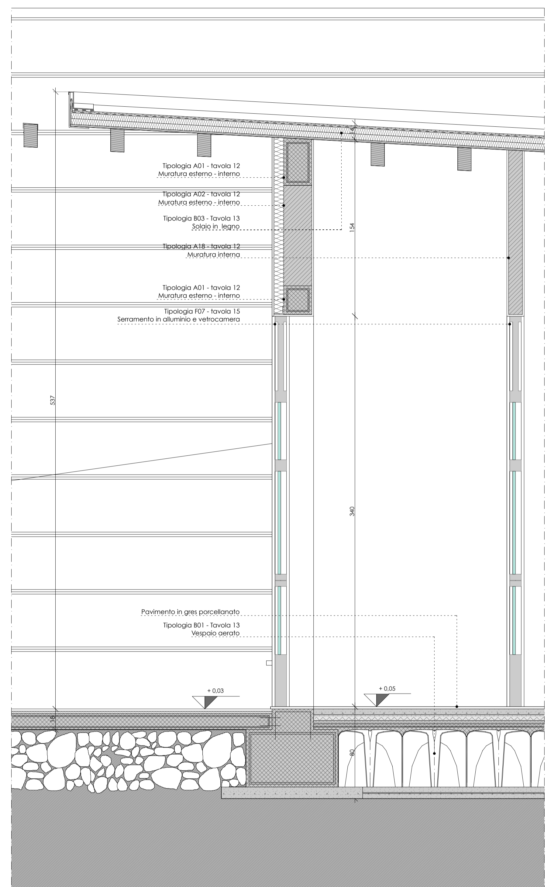
SEZIONE F-F
