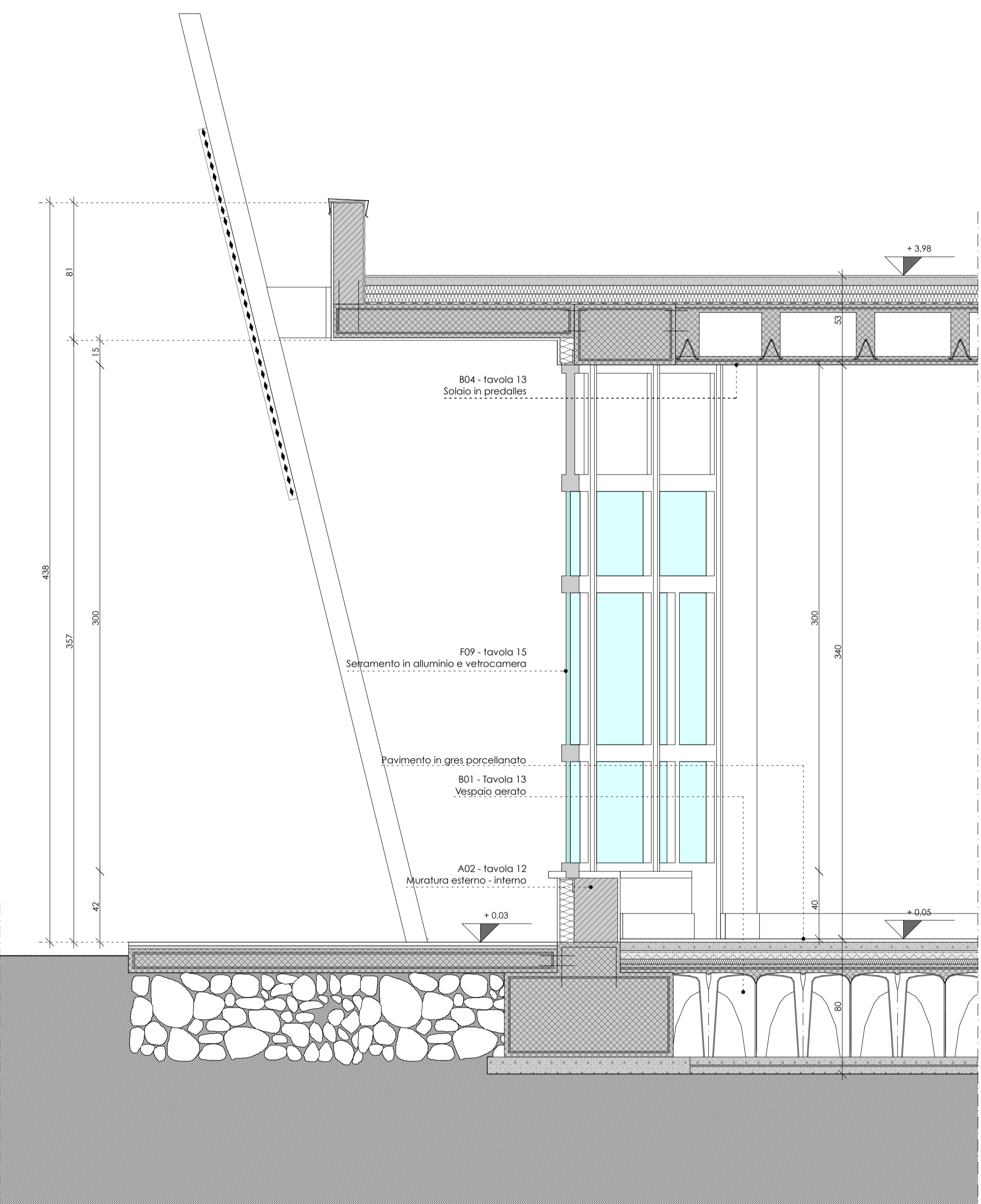
SEZIONE E-E
