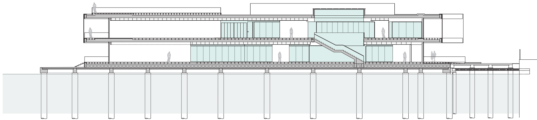
0 1 5m LONGITUDINAL SECTION
