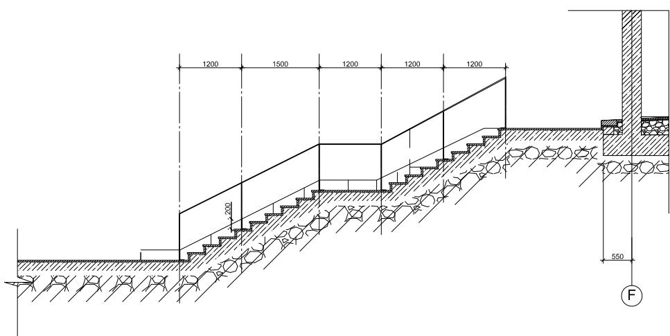
ქიბა 4 -ის შრილი. შ. 1:50
