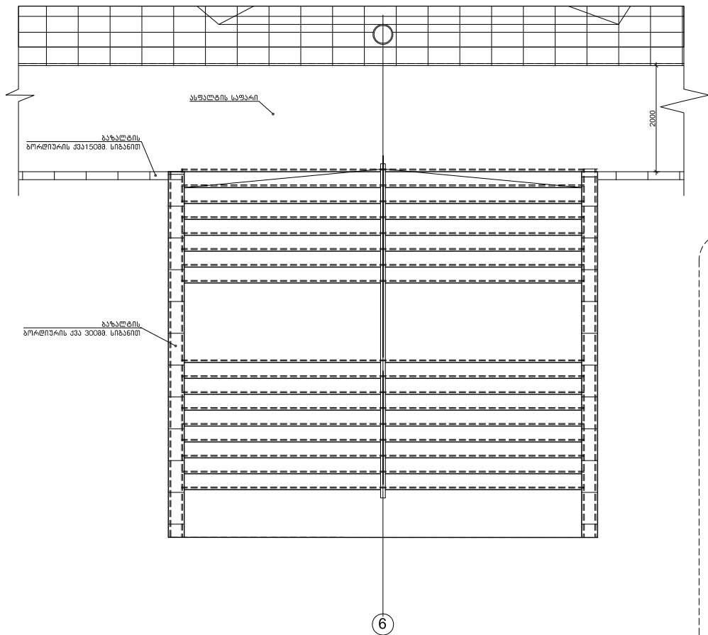
ქიბა 4 -ის ბაზა. შ. 1:50
