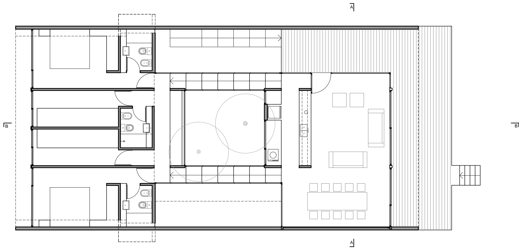
CASA S+J - PLANTA ALTA
