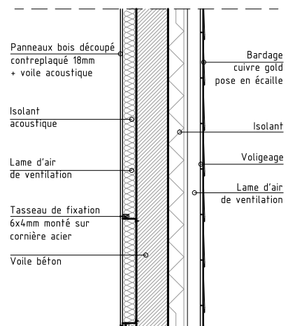
détail du complexe de façade de la salle échelle 1/50e
