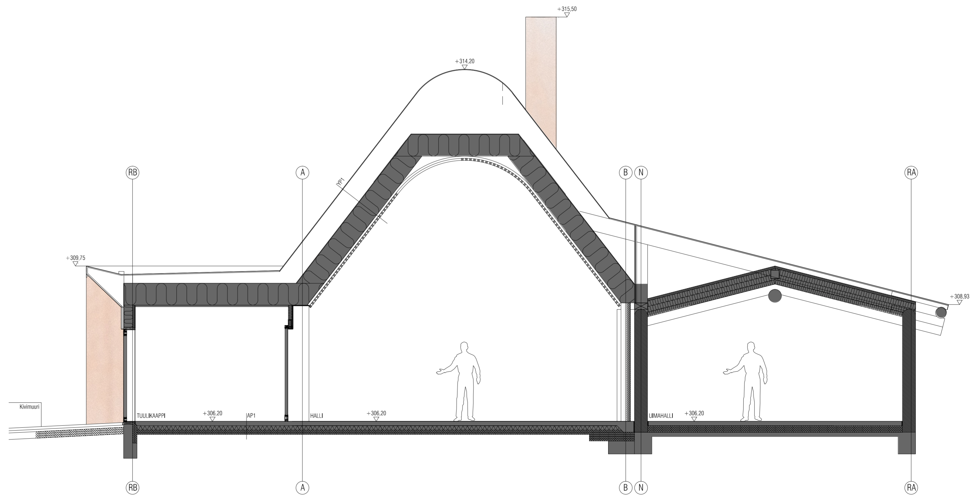
LEIKKAUS B-B 1:50
