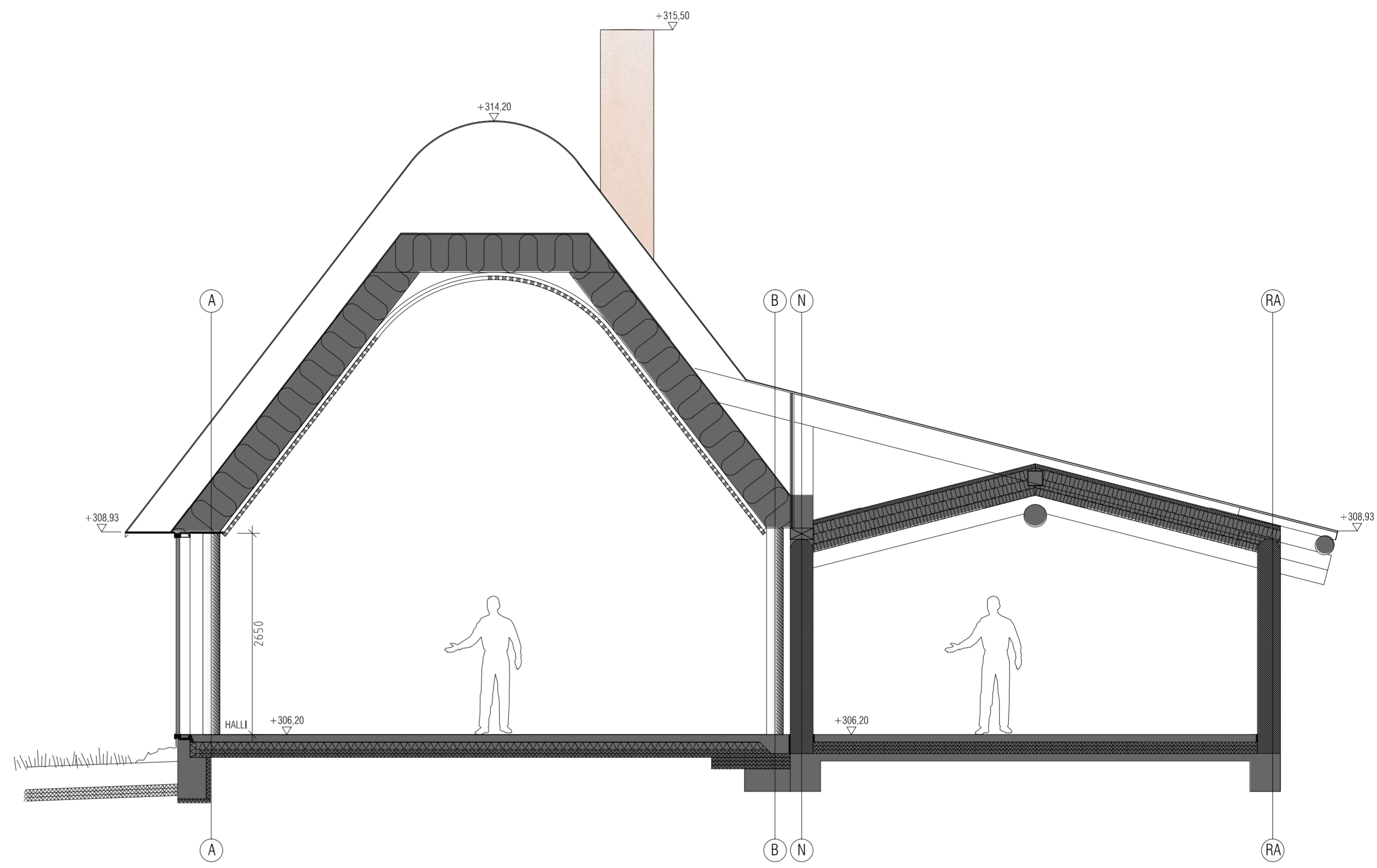
LEIKKAUS A-A 1:50
