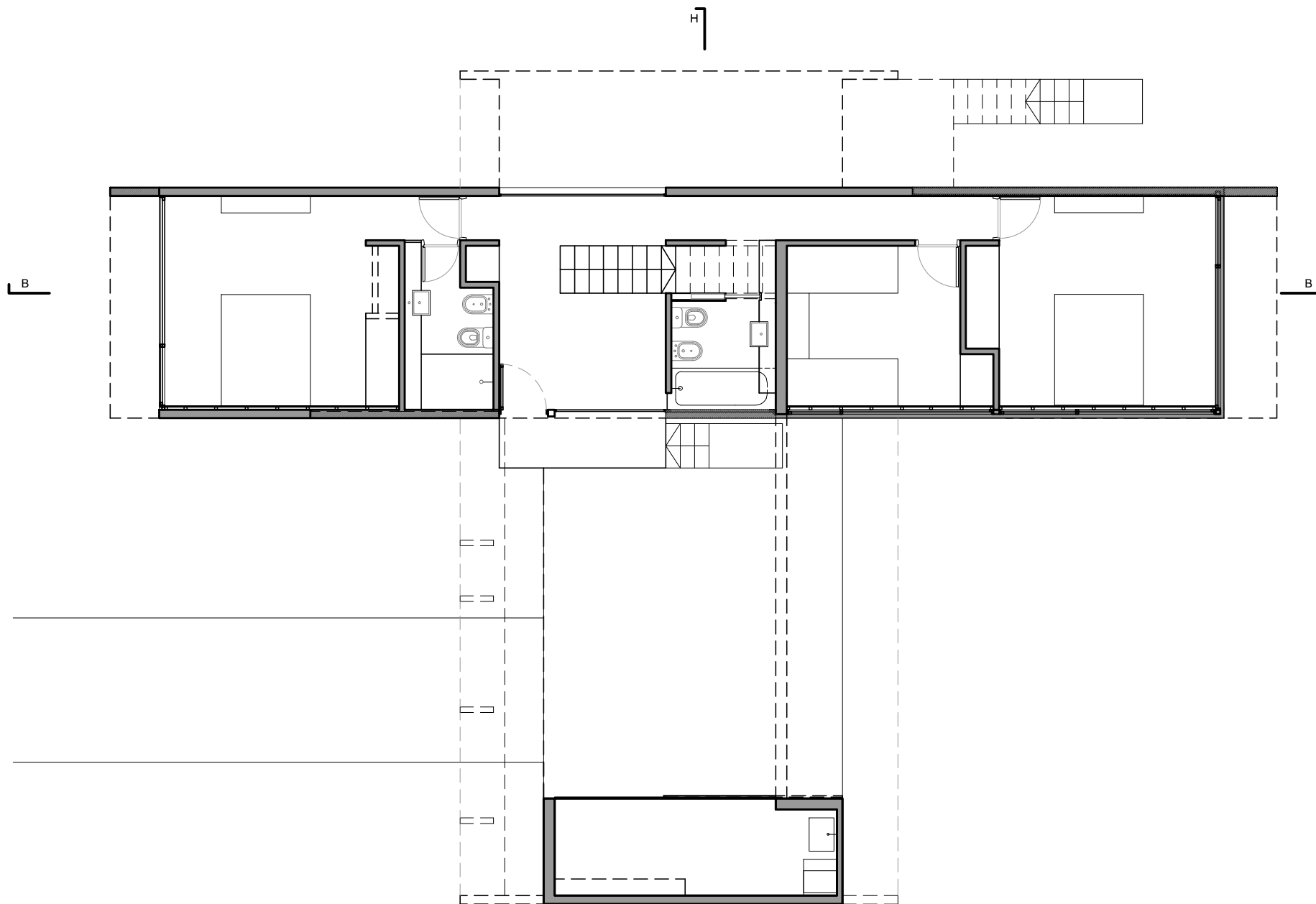
CASA GOLF - PLANTA BAJA
