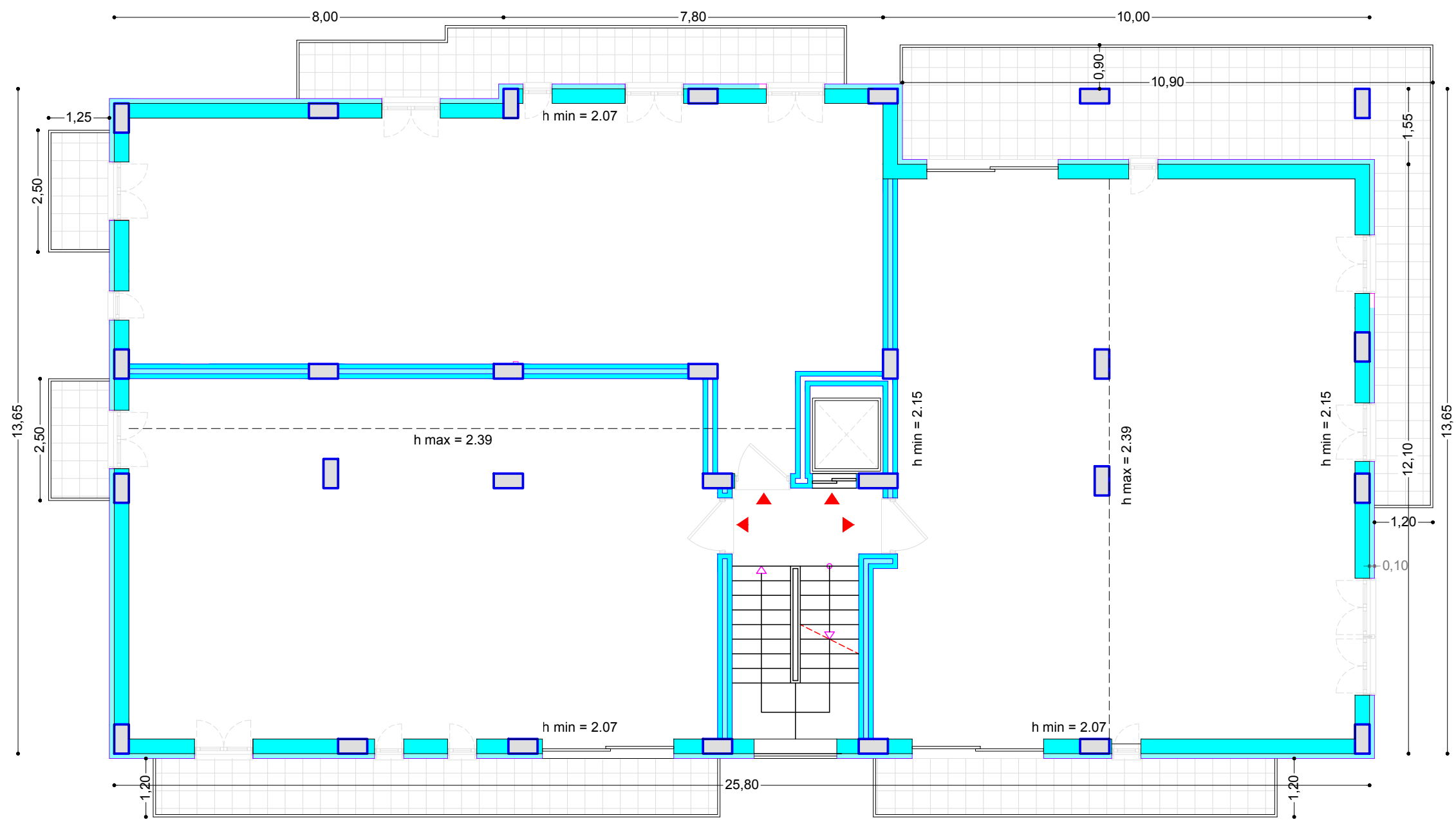
PIANTA PIANO SOTTOTETTO
