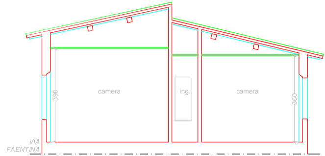
SEZIONE A-A
