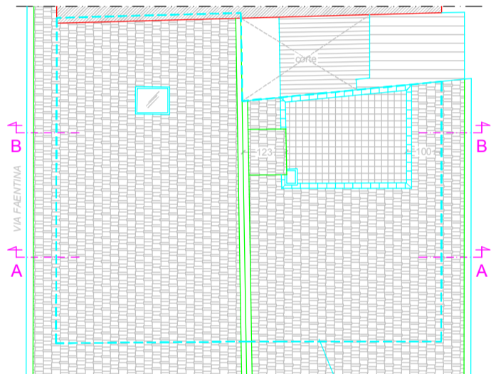
PIANTA COPERTURA
