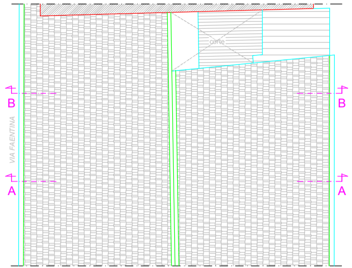
PIANTA COPERTURA
