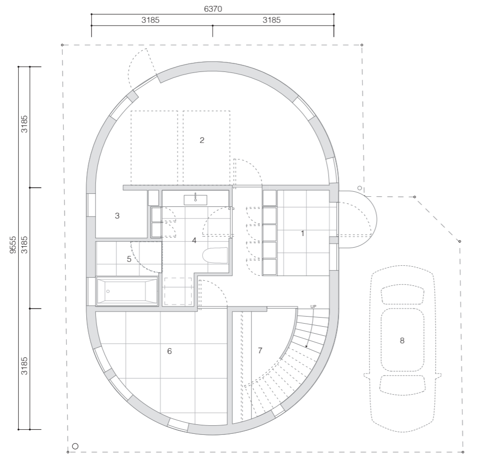
1F plan 1:100
