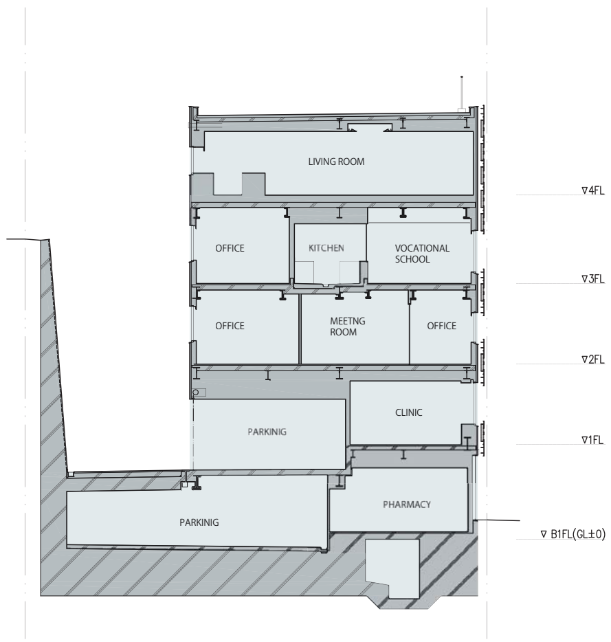
A-A' SECTION
