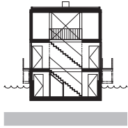
doorsnede A
