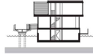
doorsnede B
