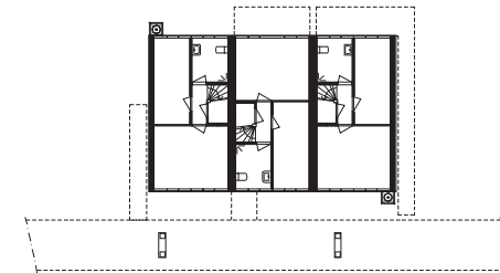
laag -01
