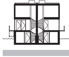
doorsnede A
