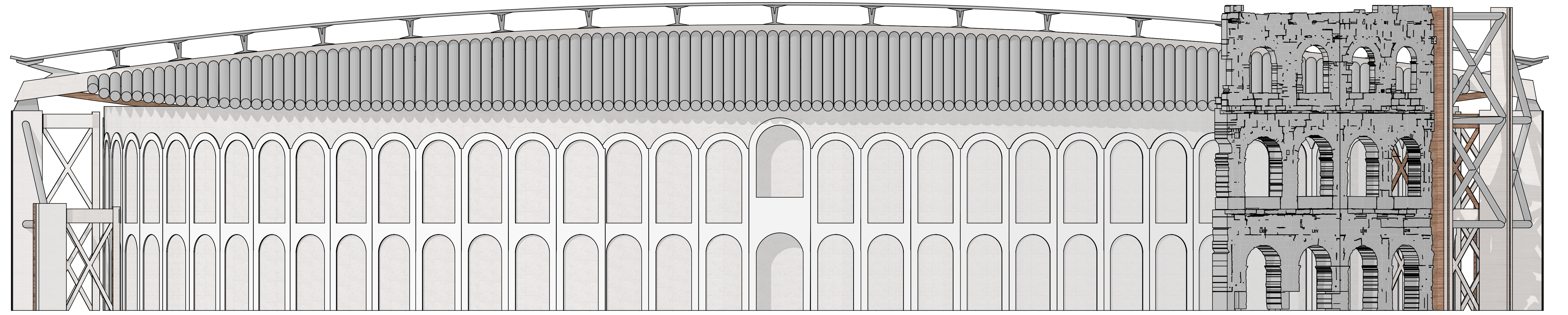
PROSPETTO NORD (VIA DIETRO ANFITEATRO)
