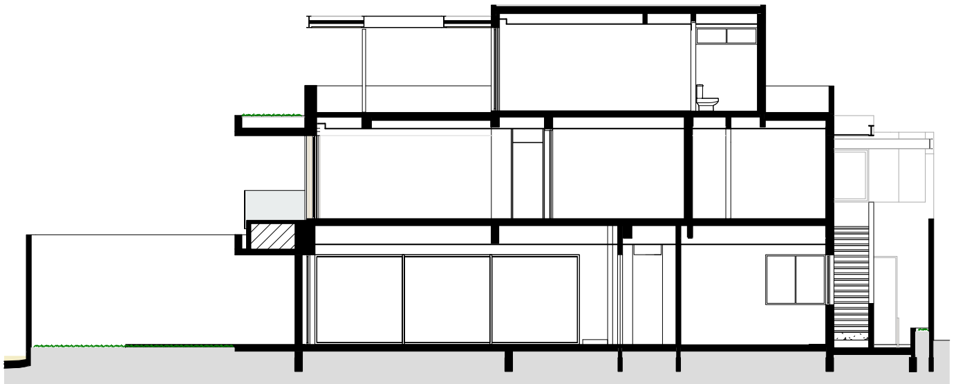
CORTE B-B
