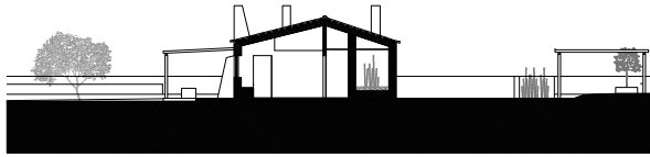
CORTE F
