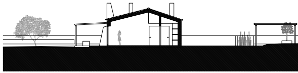
CORTE E
