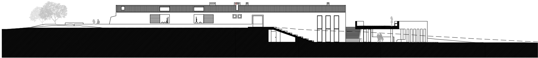
CORTE A
