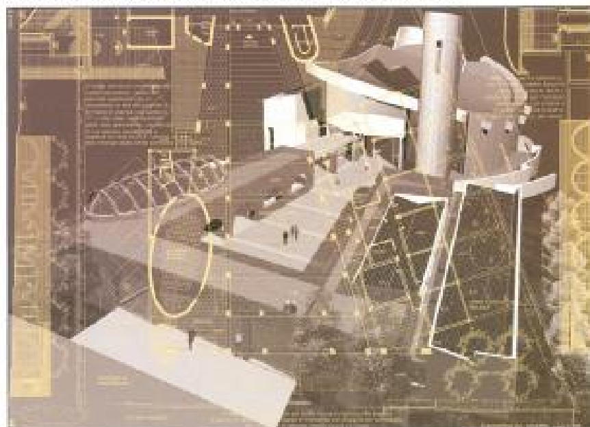
Tavola di progetto. Sulla parte sinistra è posta in particolare evidenza la sala polivalente dalla caratteristica copertura a carena rovesciata. Sulla destra, si nota il complesso articolarsi del porticato che dà adito alle aule.
