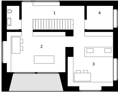
EBENE 0 livello 0
