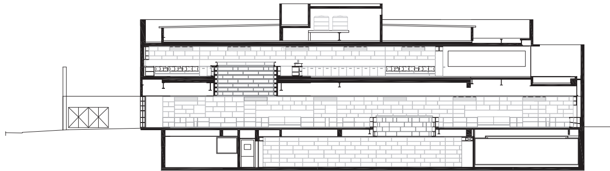
LONGITUDINAL SECTION
