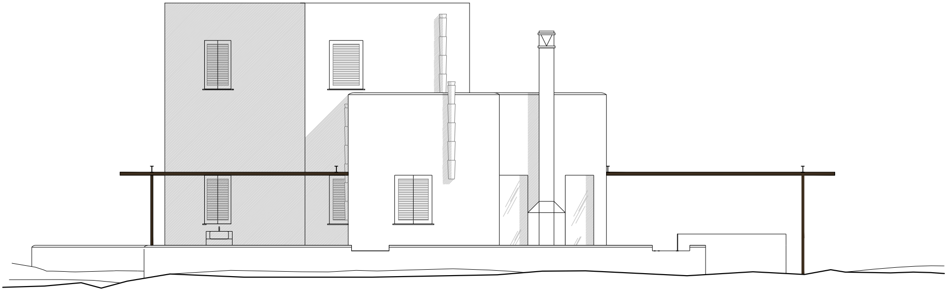
prospetto ovest
