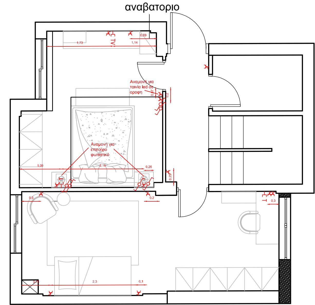
ΗΛΕΚΤΡΟΛΟΓΙΚΟ 2nd FLOOR
