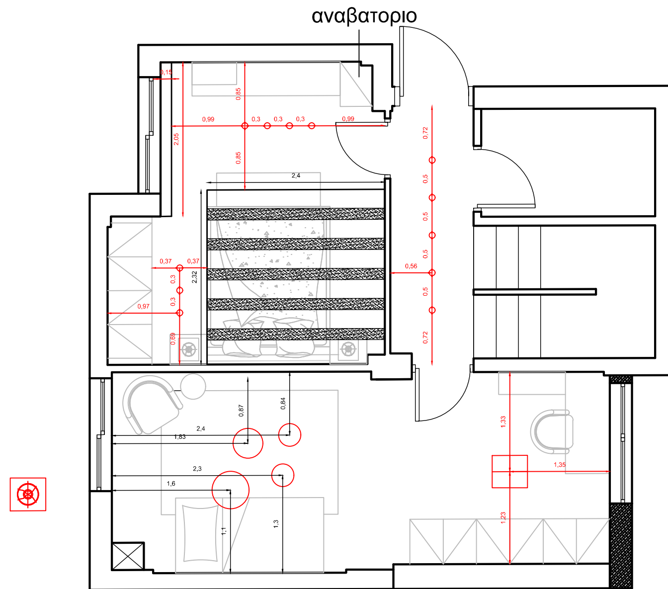
ΑΝΟΠΗ 2nd FLOOR
