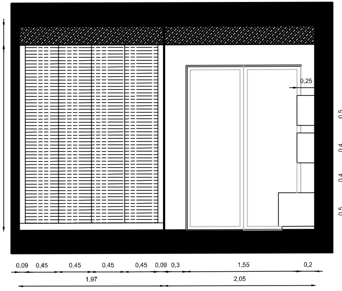
ΑΝΟΠΗ 2nd FLOOR
