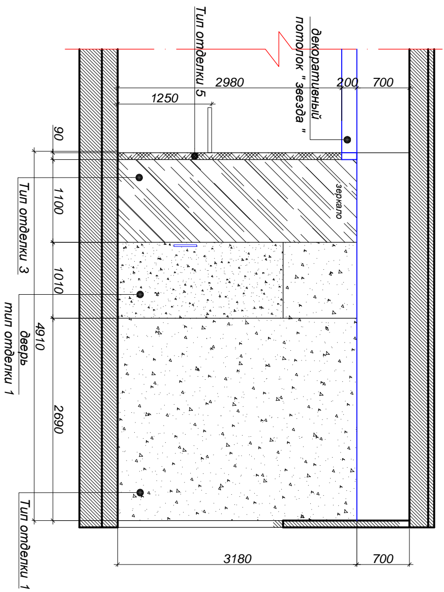
Развертка 1-2 М 1:50
