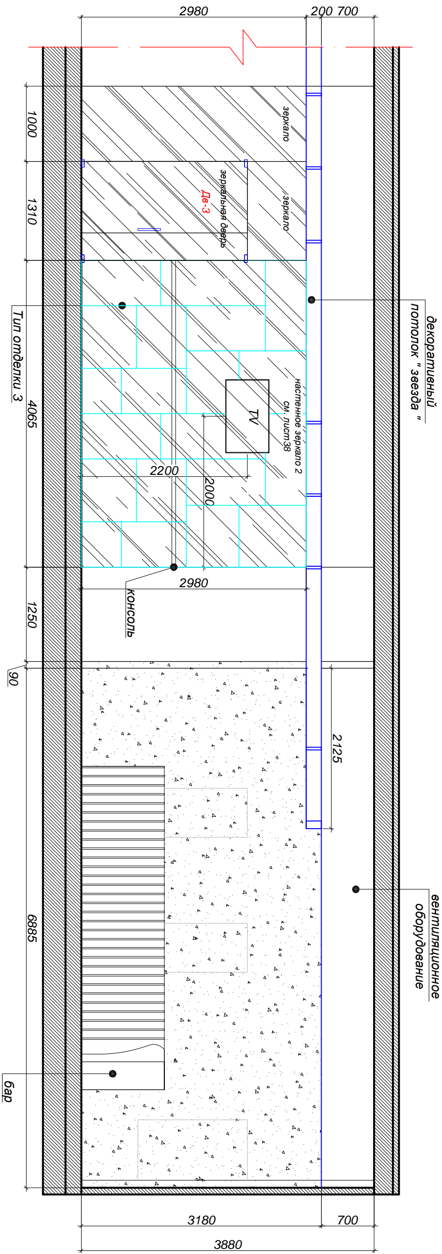
Развертка К-Л М 1:50
