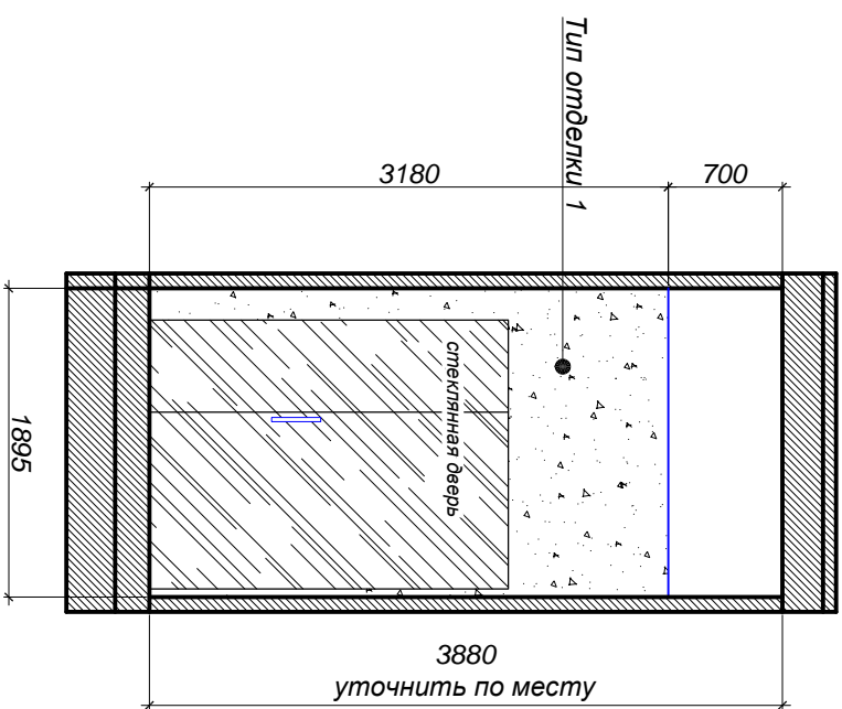
Развертка 2-3 М 1:50
