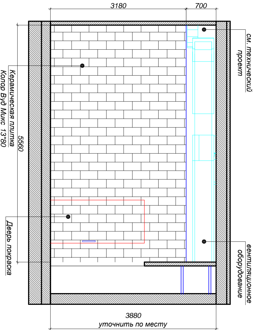
Развертка Л-А М 1:50
