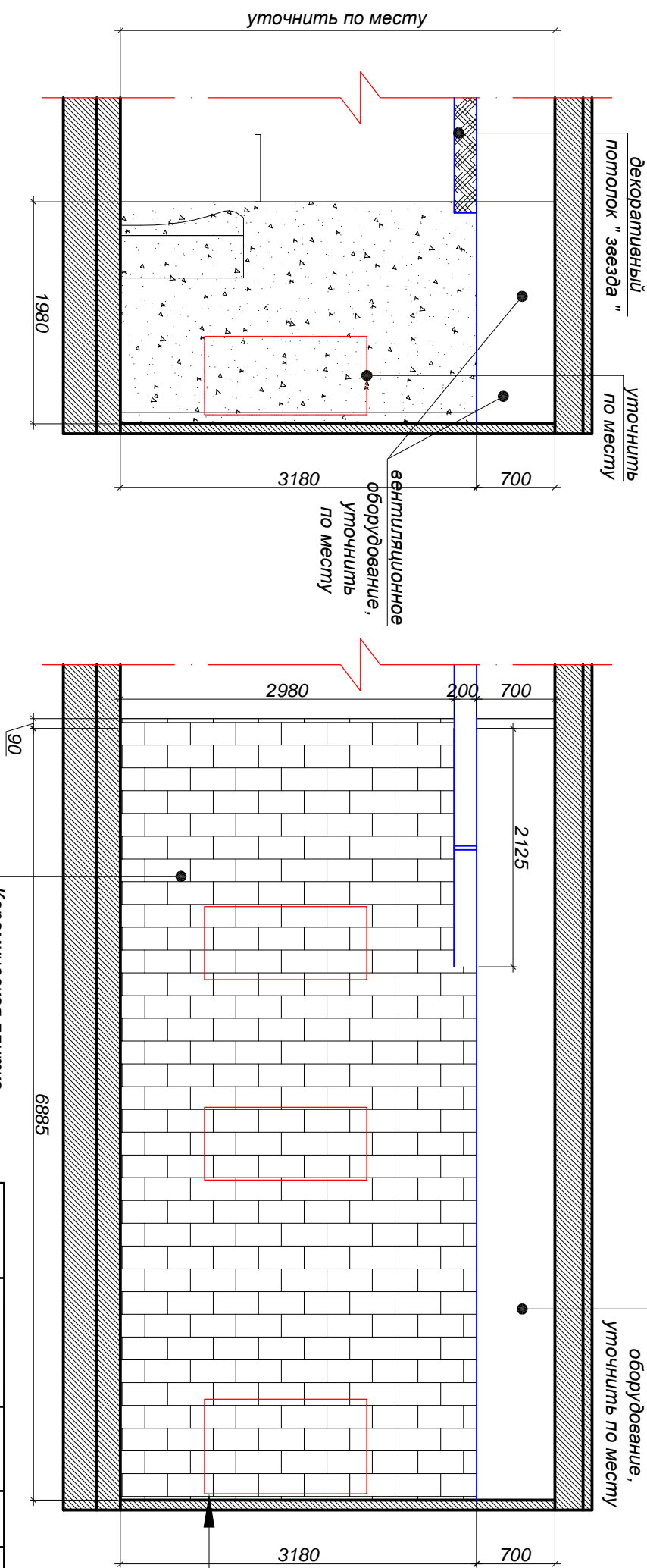
Развертка К-Л М 1:50
