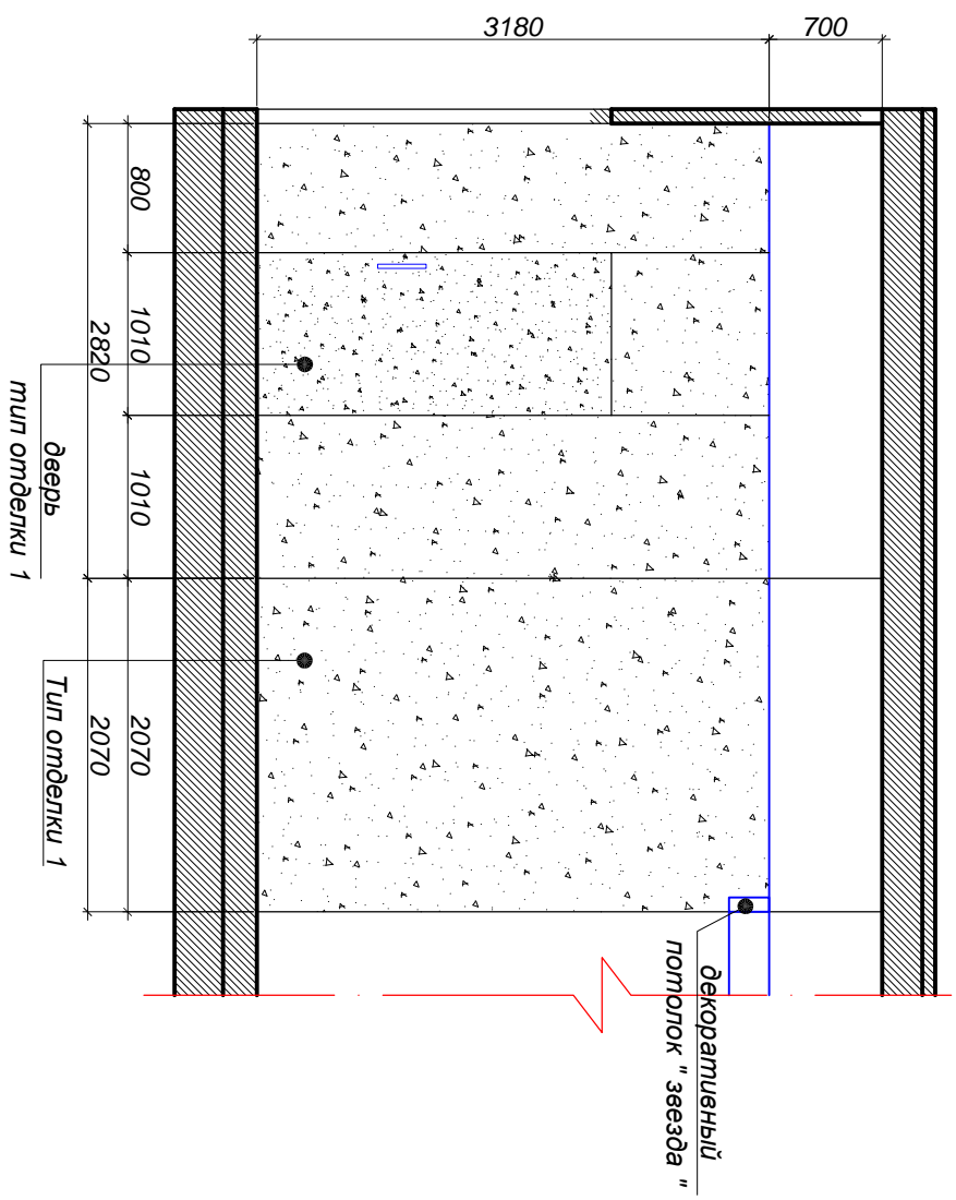
Развертка 3-4 М 1:50
