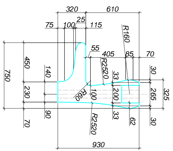
Сечение 1-1 М 1:25
