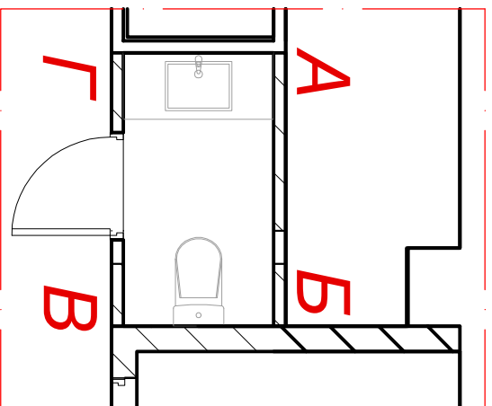
План-схема санузла М 1:50
