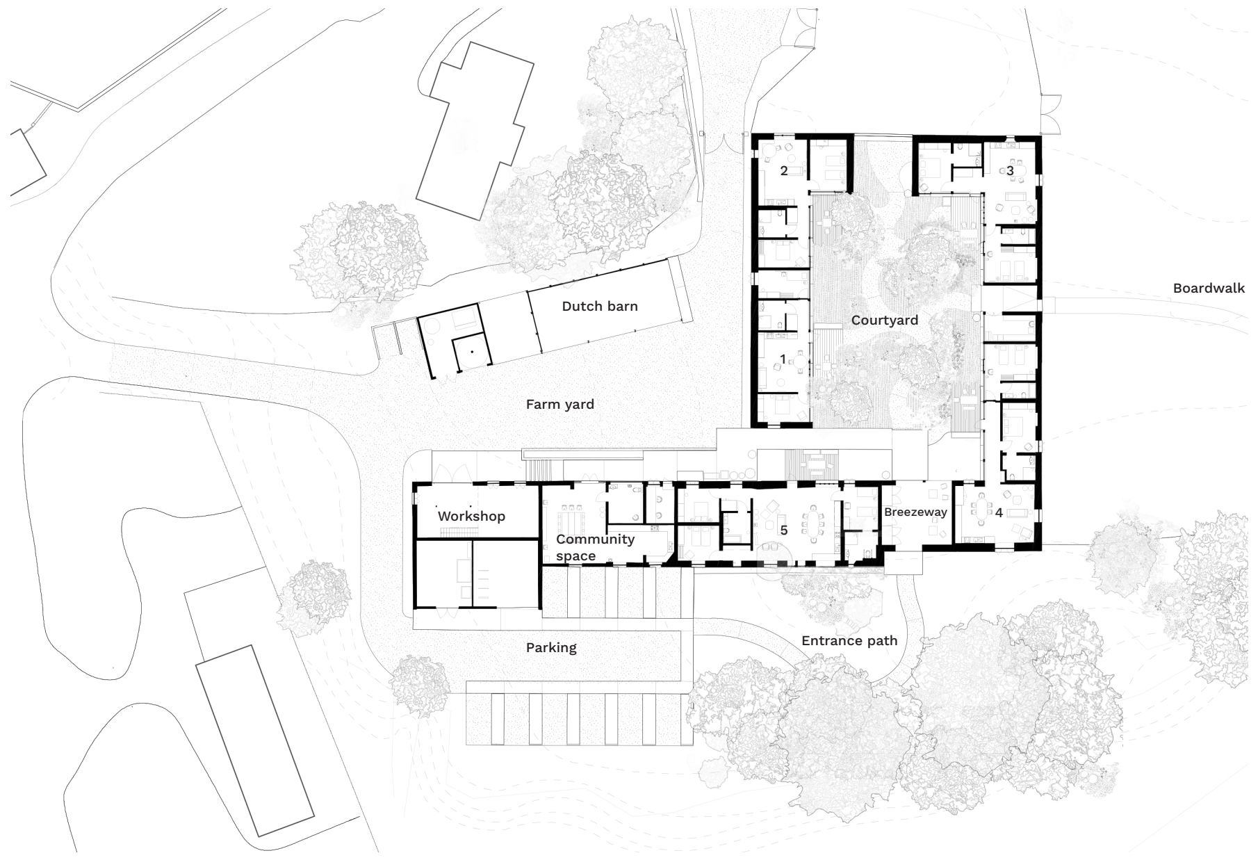
Plan 1:500 @ A3
