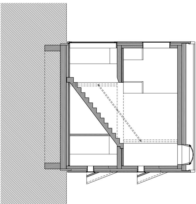
querschnitt
