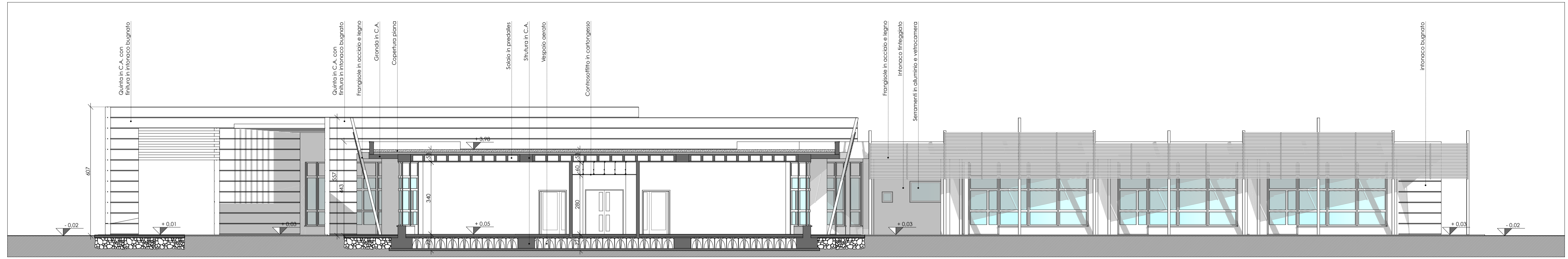
SEZIONE A-A
