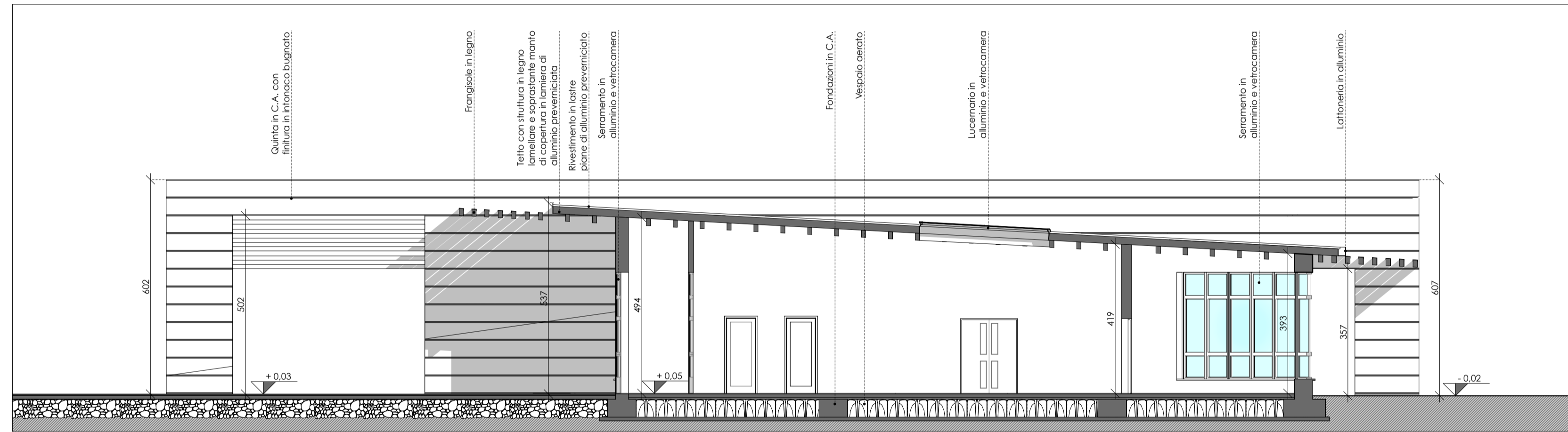
SEZIONE B-B
