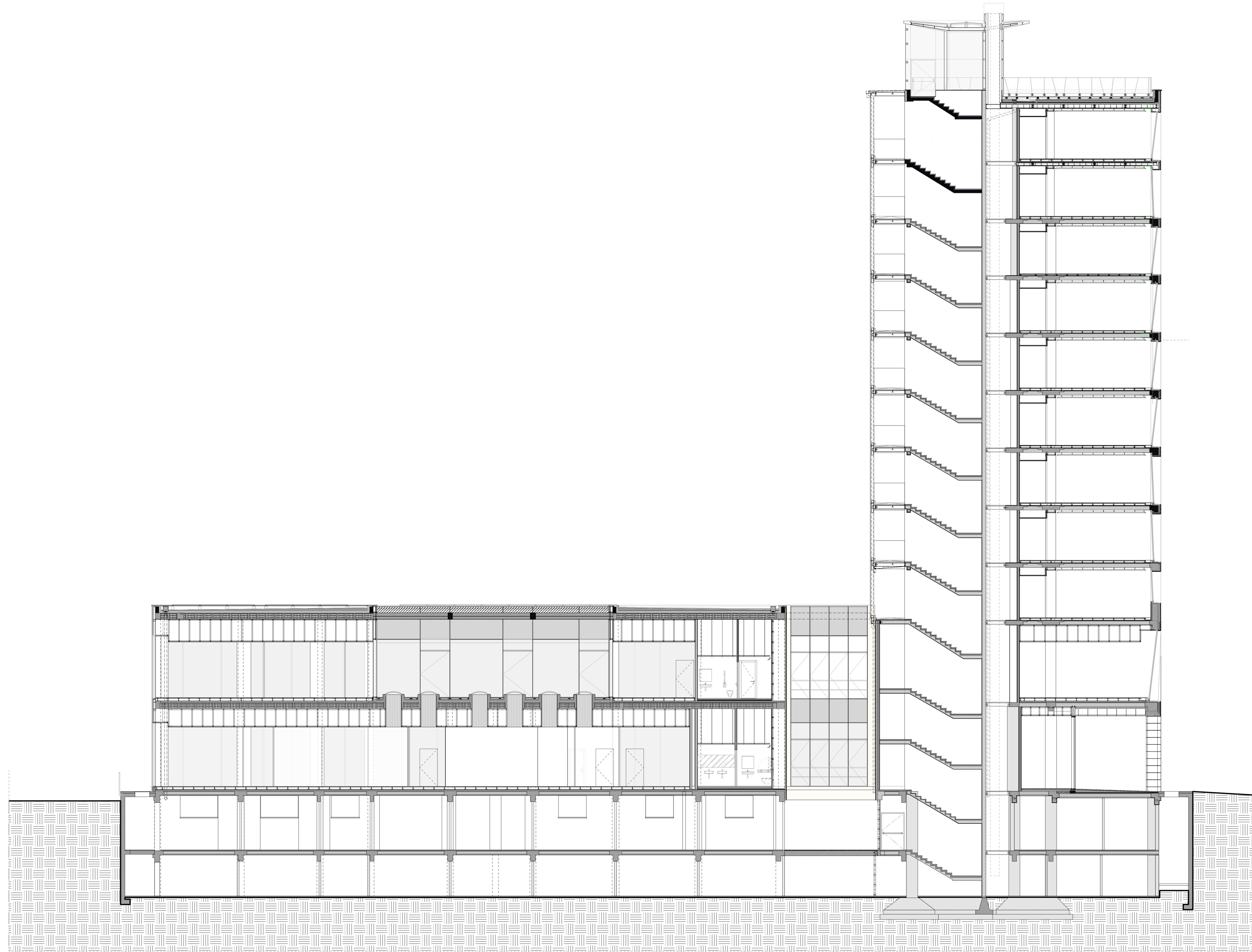
sezione A-A progetto_scala 1:100
