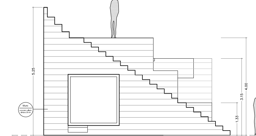
Fachada Sur cuarto Master
