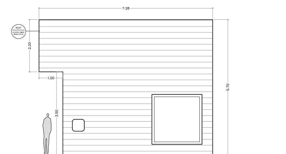
Fachada Este Cuarto entrada
