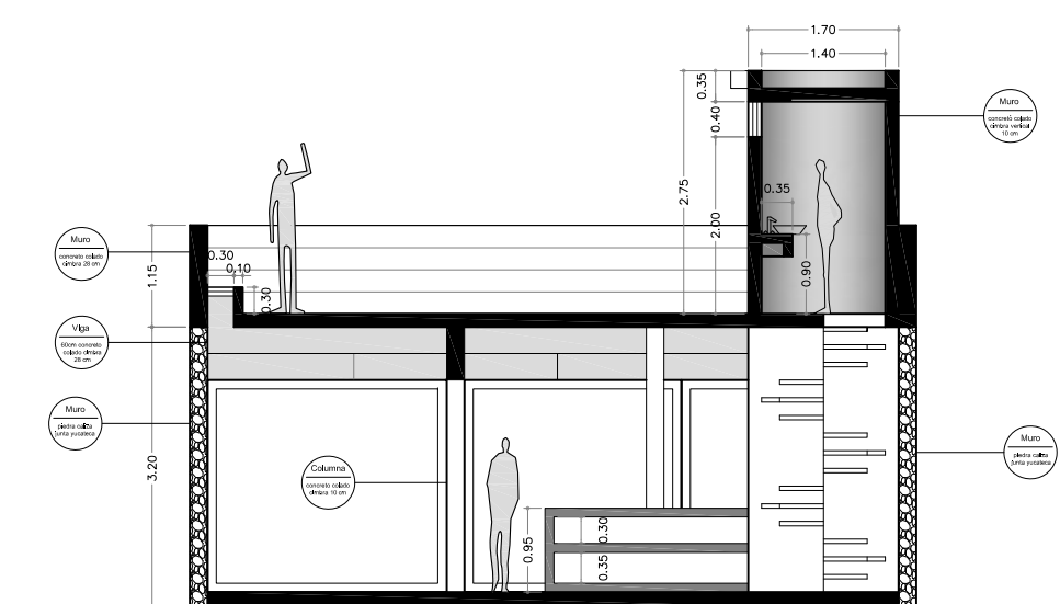
Corte Transversal Estanda
