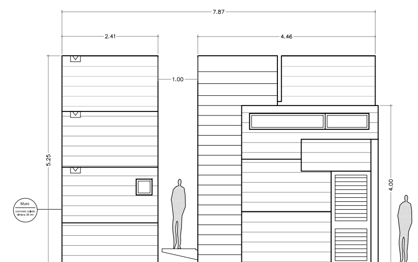
Fachada Este cuarto y baño Master
