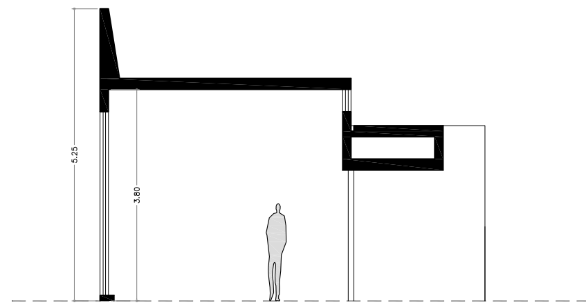
Corte transversal cuarto Master
