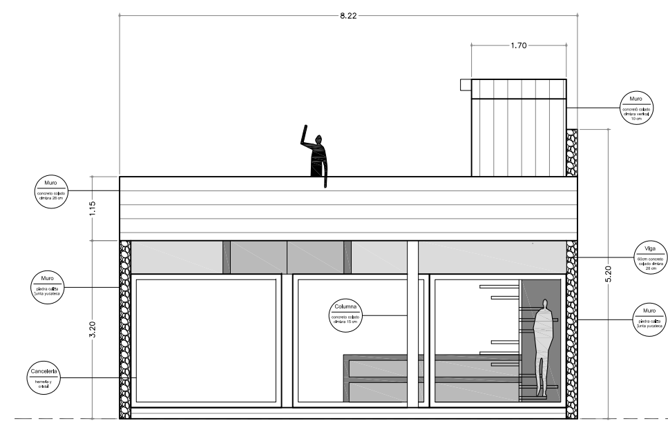
Fachada Este Estanda
