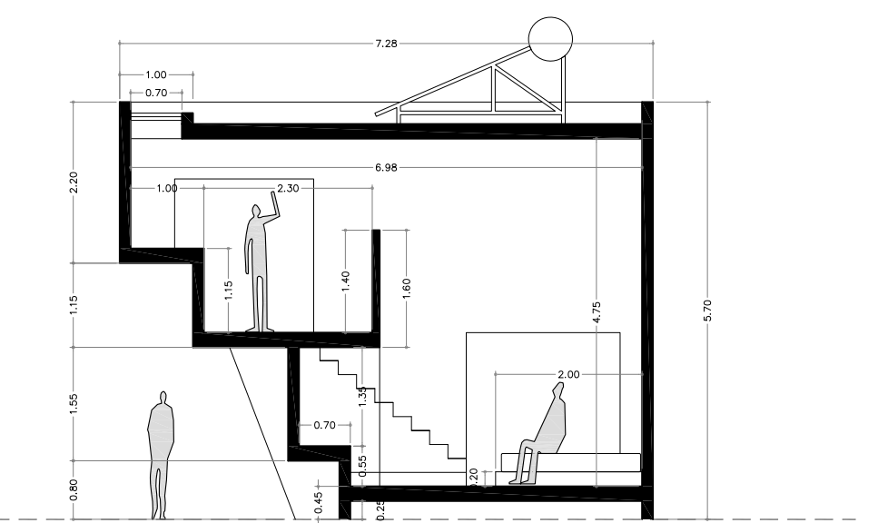
Corte transversal Cuarto entrada
