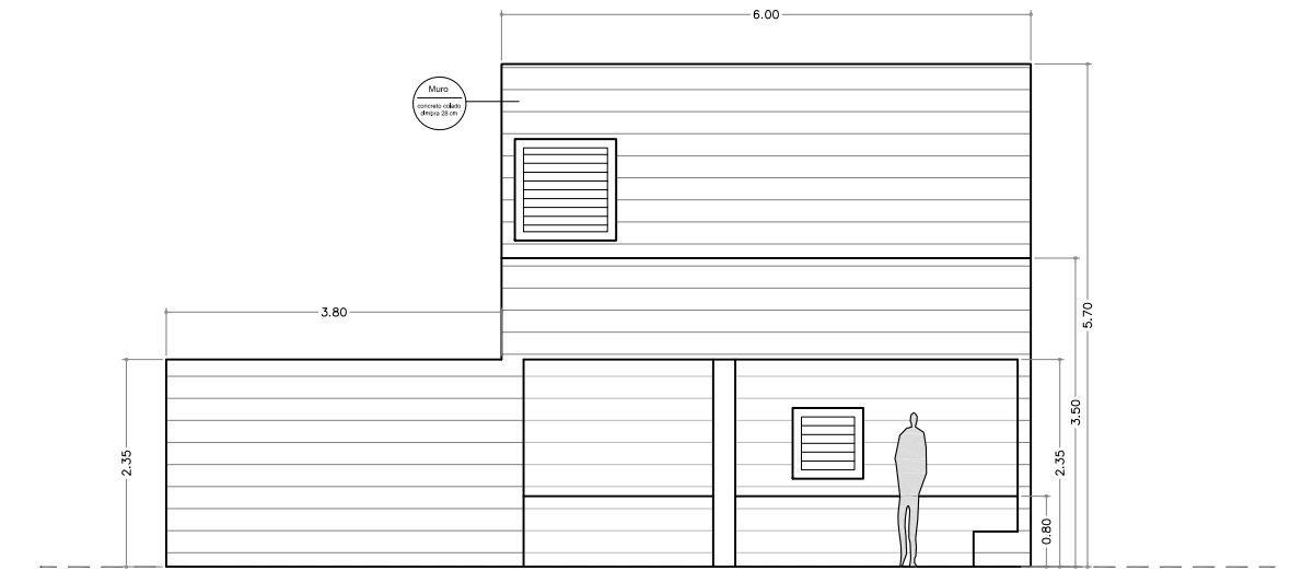
Fachada Sur Cuarto entrada
