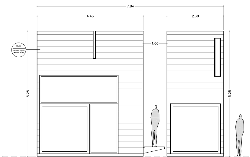
Fachada Oeste cuarto y baño Master
