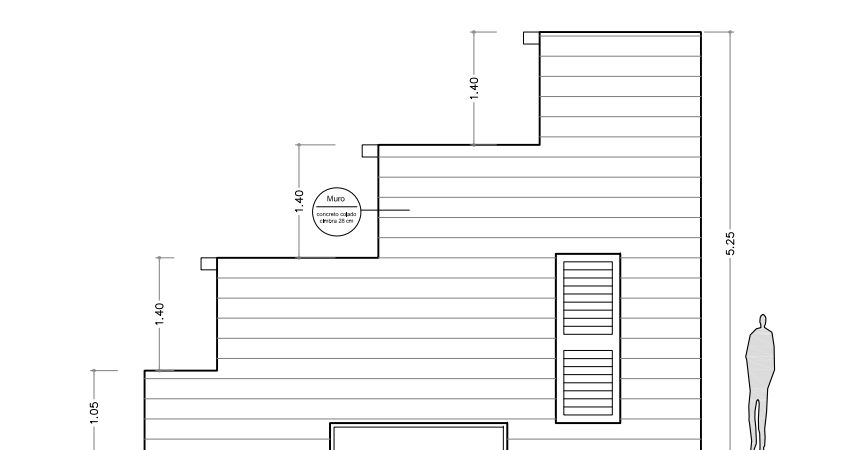
Fachada Norte baño Master
