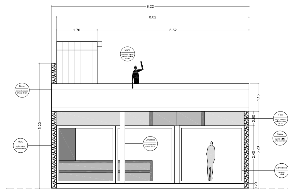
Fachada Oeste Estanda
