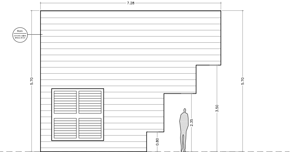
Fachada Oeste Cuarto entrada
