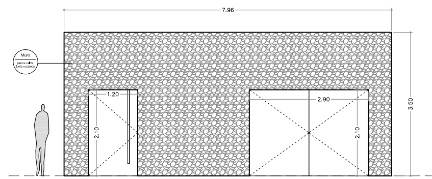
Fachada a la calle
