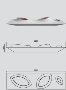
umywalka / washbasin #022222
