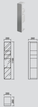
szafka / cupboard #021229
