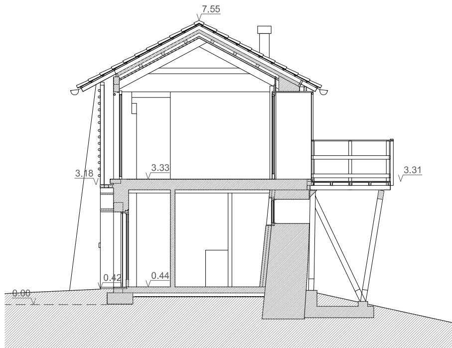
SEZIONE B-B
