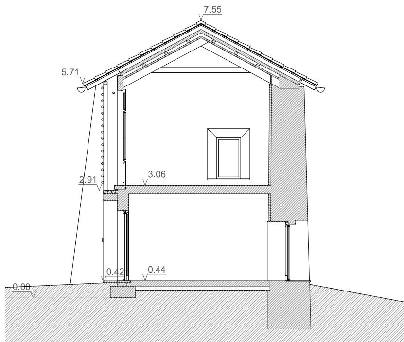
SEZIONE A-A
