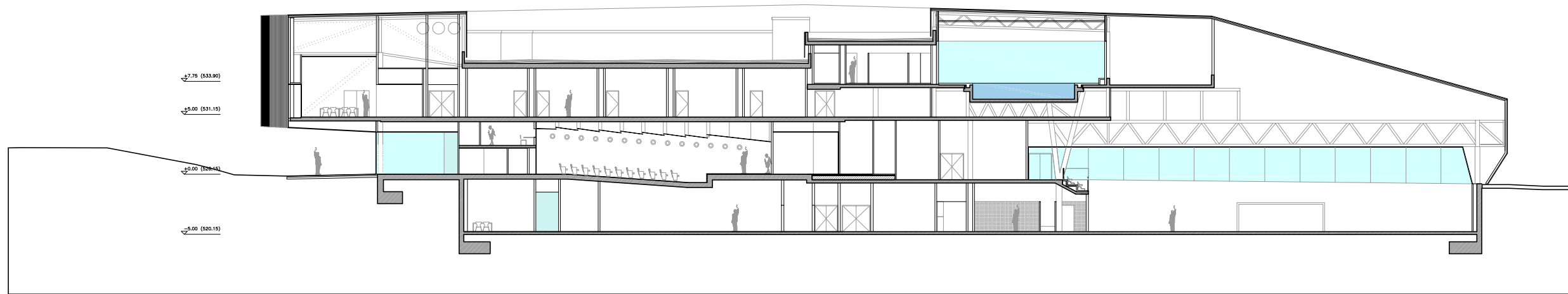
SECCION S5
