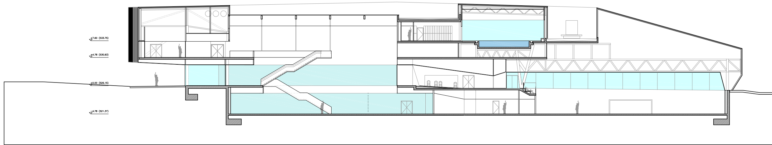
SECCION S4
