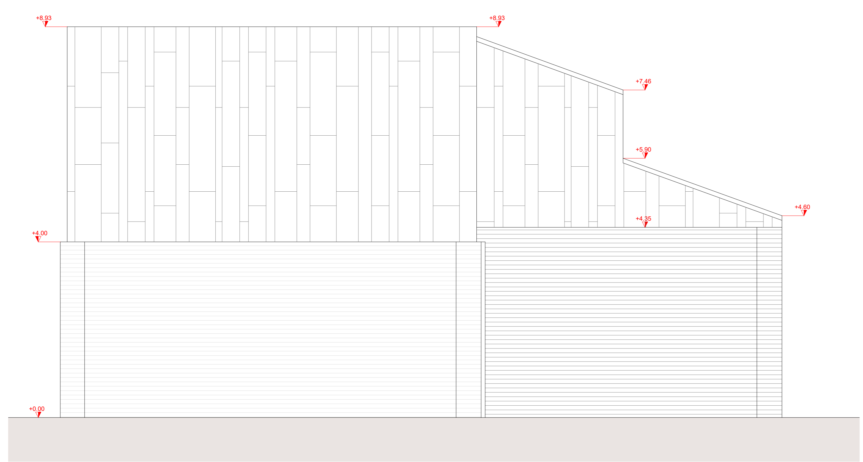
PROSPETTO NORD
